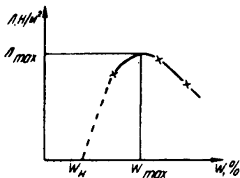
Рис. 1. Зависимость липкости грунта от его влажности
