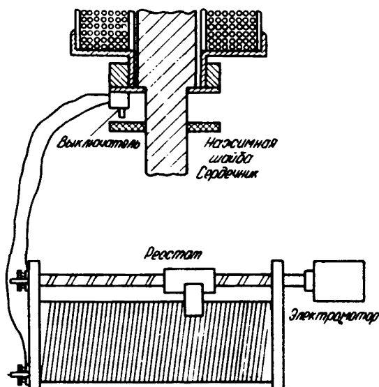
Рис. 4. Устройство для автоматической регистрации момента отрыва штампа от грунта в приборе УИЛ-2
