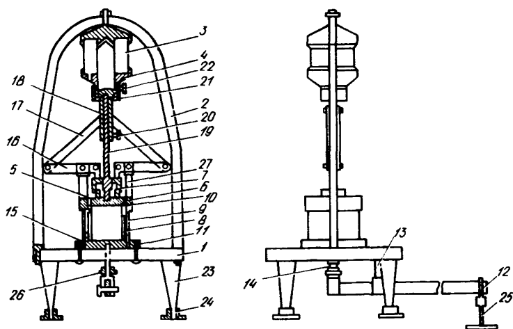
Рис. 2. Лабораторный прибор (устройство) для измерения липкости грунтов УИЛ-2
