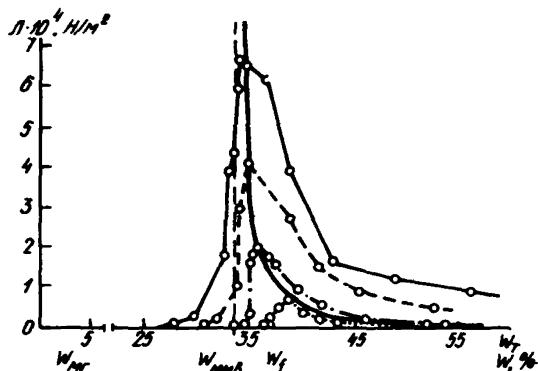
Рис. 9. Зависимость липкости глинистого грунта от его влажности при различных значениях предварительной прижимающей нагрузки
