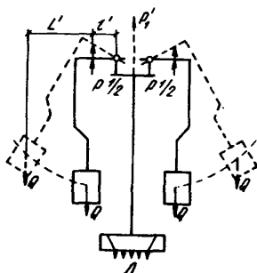
Рис. 8. Схема передачи отрывающего усилия в приборе ППЛ-1
