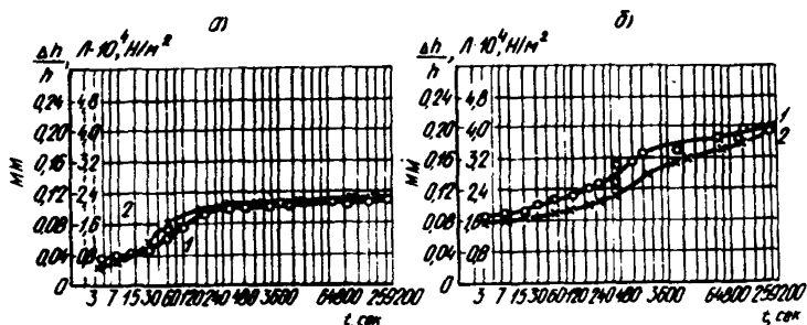
Рис. 10. Зависимость липкости (кривая 1) а – каолинитовой глины; б – монтмориллонитовой глины от времени действия предварительной прижимающей нагрузки; 2 – кривые консолидации тех же глин при давлении 0,3 МПа
