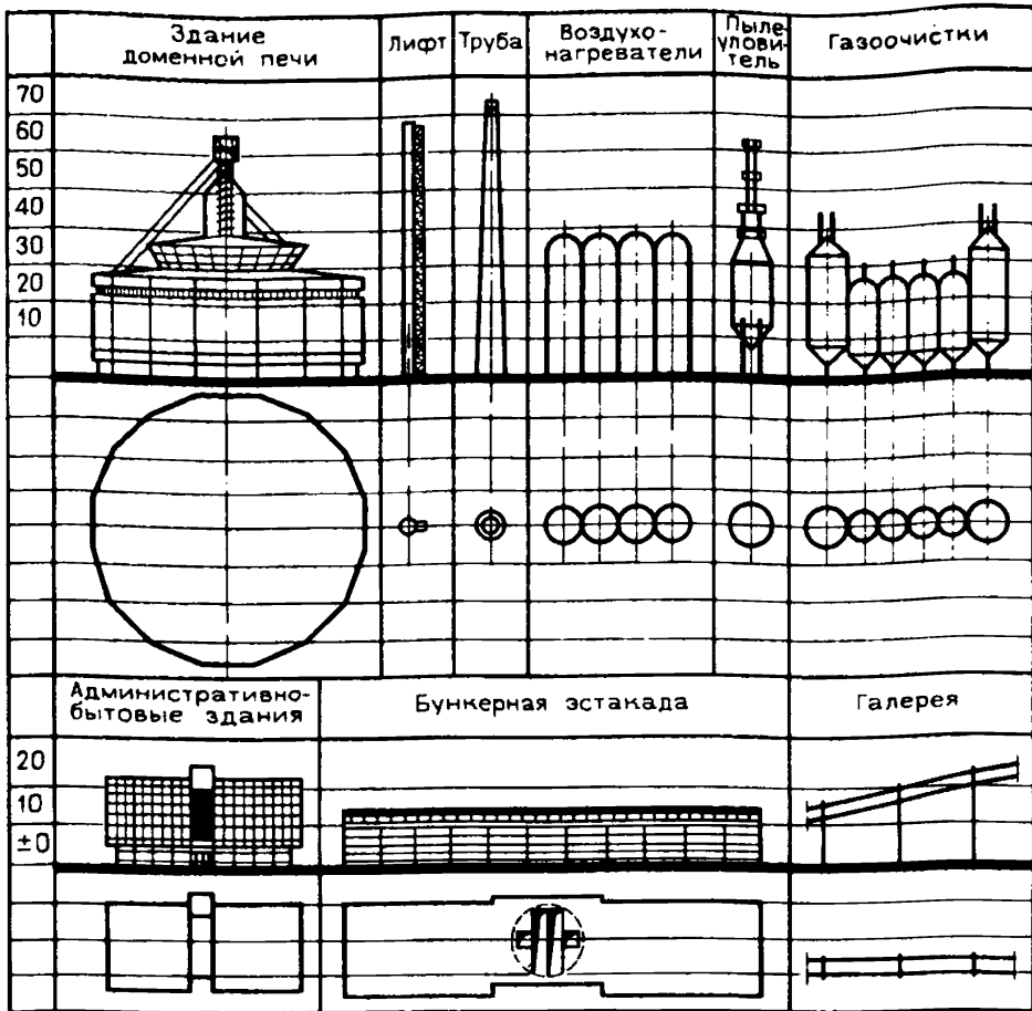
Рис. 53. Основные элементы комплекса доменной печи
