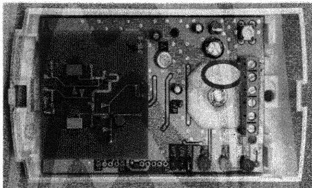
Рисунок 23 – Переключатель «Р» на плате
