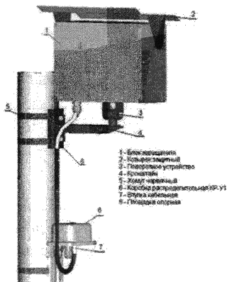
Рисунок 33 - Внешний вид блока извещателя «Радий-7»
