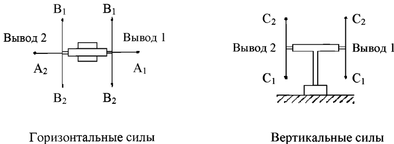
а) Статические нагрузки на выключатель
