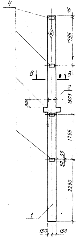
Разрез В-В
