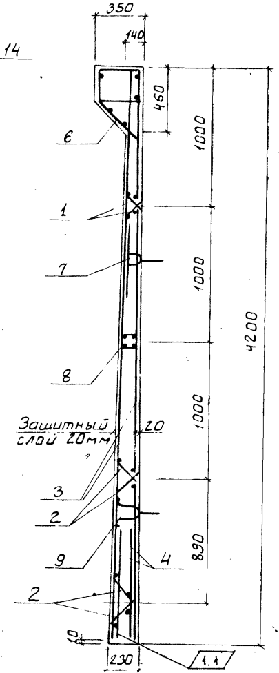
А-А (армирование)
