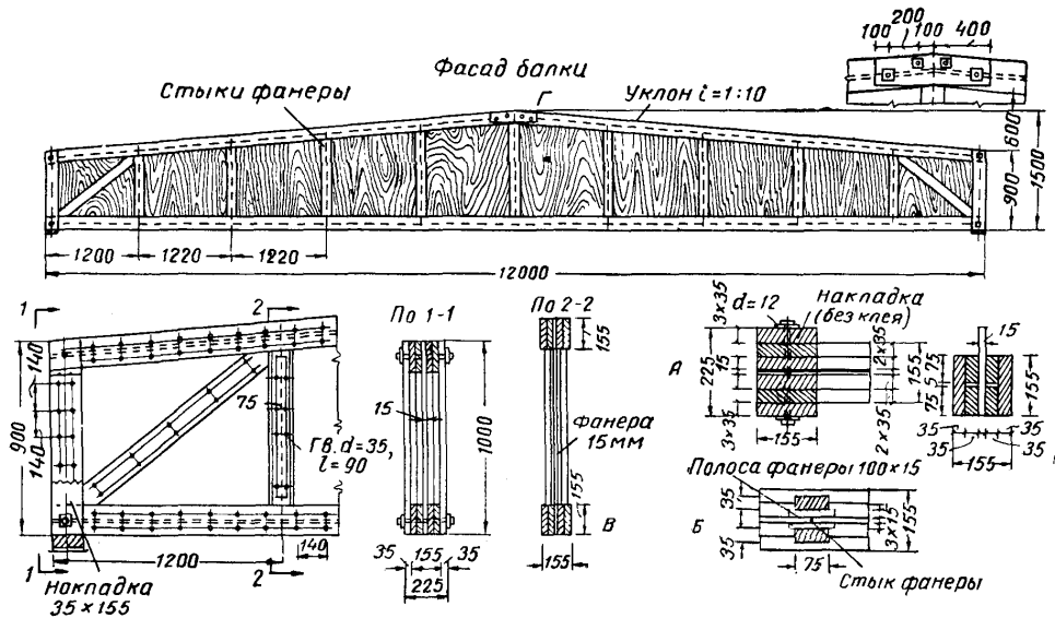
Рис. 9. Двухтавовая балка с фанерной стенкой
