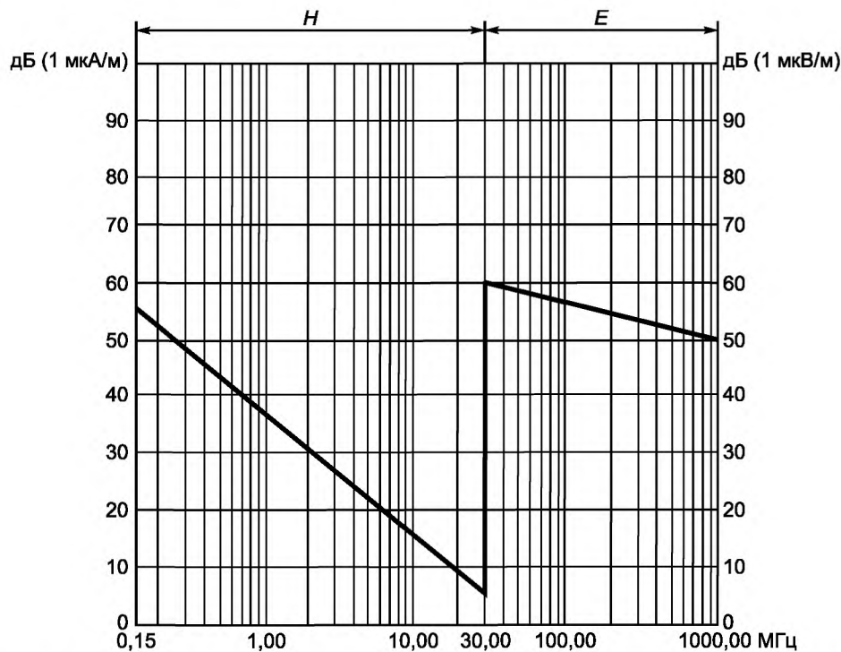
Рисунок 2 — Нормы напряженности поля электромагнитных помех (квазипиковые значения) от тяговых подстанций
