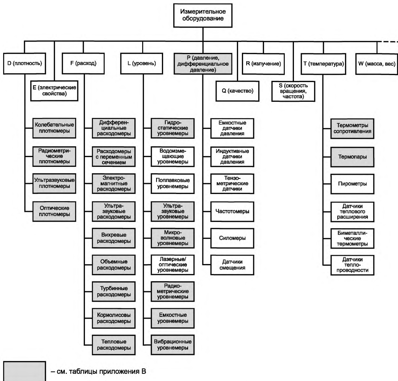
Рисунок 1 — Схема классификации производственного измерительного оборудования
