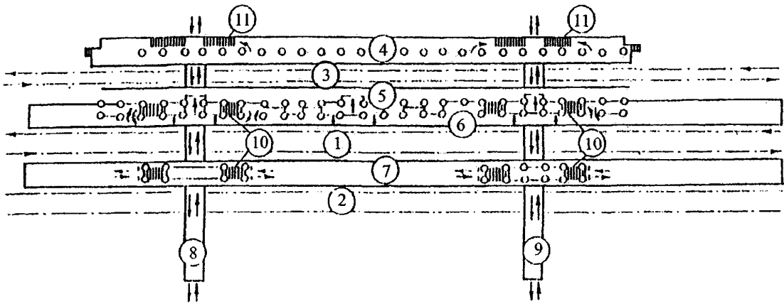
1, 2 – пути железнодорожной станции; 3 – пути метрополитена; 4, 5 – платформы метрополитена; 6, 7 – платформы железнодорожной станции; 8, 9 – подземные переходы, соединяющие платформы с выходом в город; 10 – лестницы, оборудованные пандусом; 11 – лестницы, оборудованные эскалатором или подъемником
