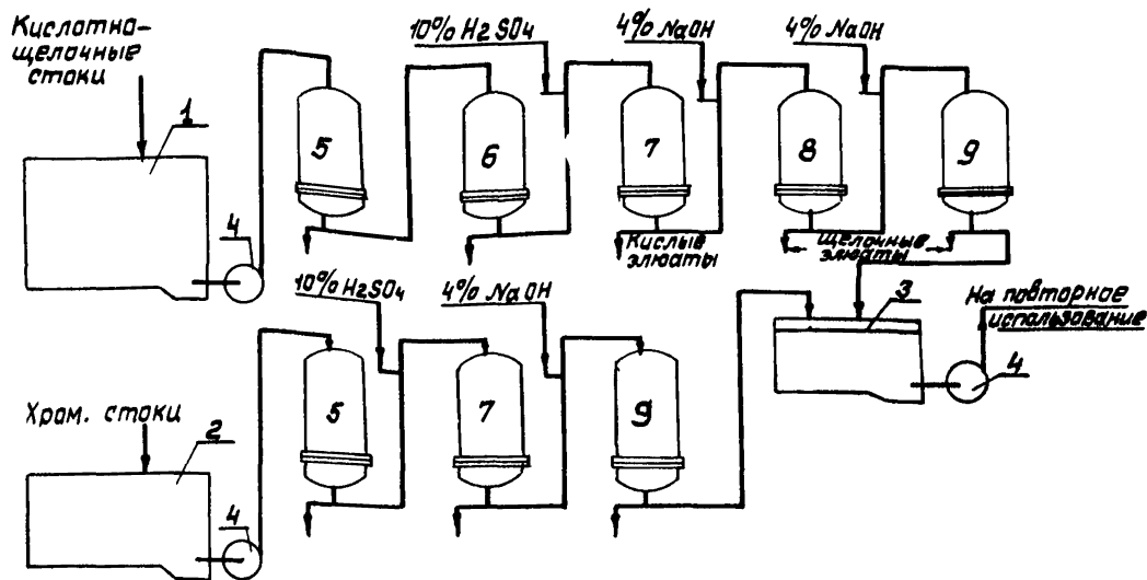
Рис.13. Принципиальная схема очистки кислотно-щелочных и хромсодержащих стоков методом ионного обмена
