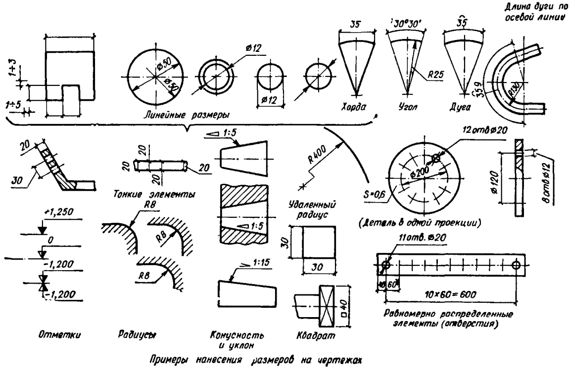
Примеры нанесения размеров на чертежах
