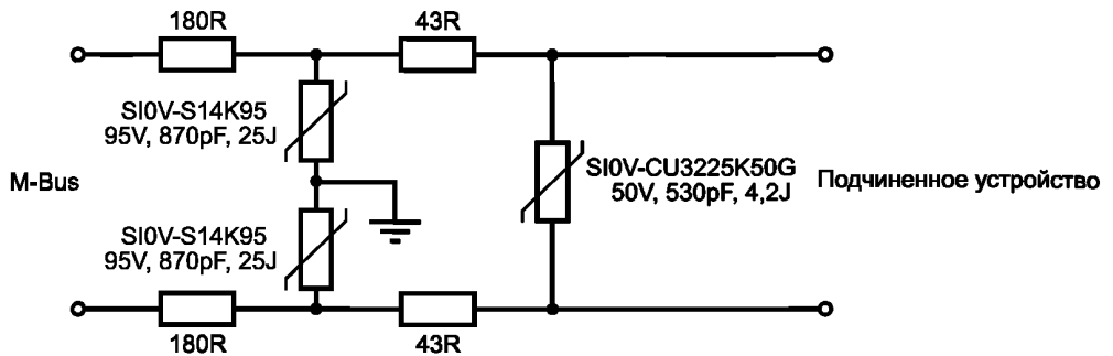
Рисунок Е.8 — С заземлением ( 100 \times 10 \text{ кВ} \times 50 \text{ мкс} или 100 \times 2 \text{ кВ} \times 1000 \text{ мкс} )
