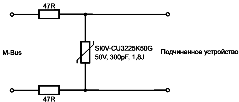
Рисунок Е.5 — Без заземления ( 100 \times 2 кВ \times 50 мкс)
