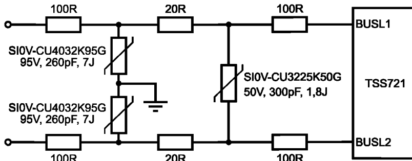
Рисунок Е.2 — С заземлением ( 100 \times 6 \text{ кВ} \times 50 \text{ мкс} )
