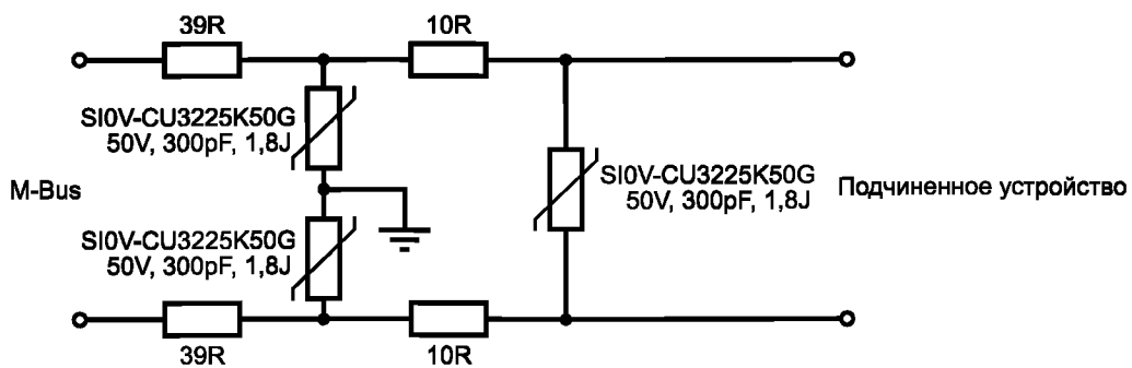
Рисунок Е.6 — С заземлением ( 100 \times 2 кВ \times 50 мкс)
