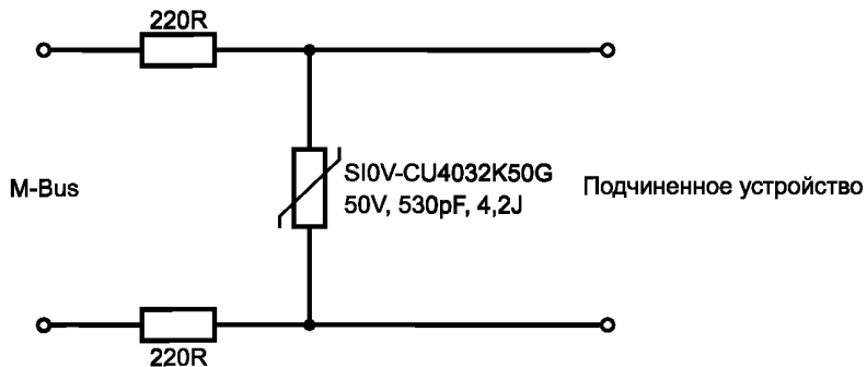
Рисунок Е.7 — Без заземления ( 100 \times 10 \text{ кВ} \times 50 \text{ мкс} или 100 \times 2 \text{ кВ} \times 1000 \text{ мкс} )
