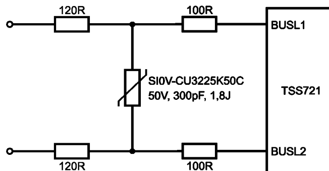
Рисунок Е.1 — Без заземления ( 100 \times 6 \text{ кВ} \times 50 \text{ мкс} )
