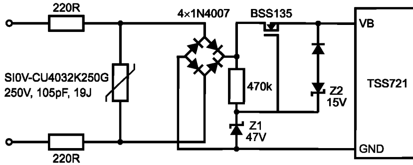
Рисунок Е.3 — Без заземления ( 100 \times 10 кВ \times 50 мкс, макс. 250 Vrms (среднеквадратичное напряжение в вольтах)
