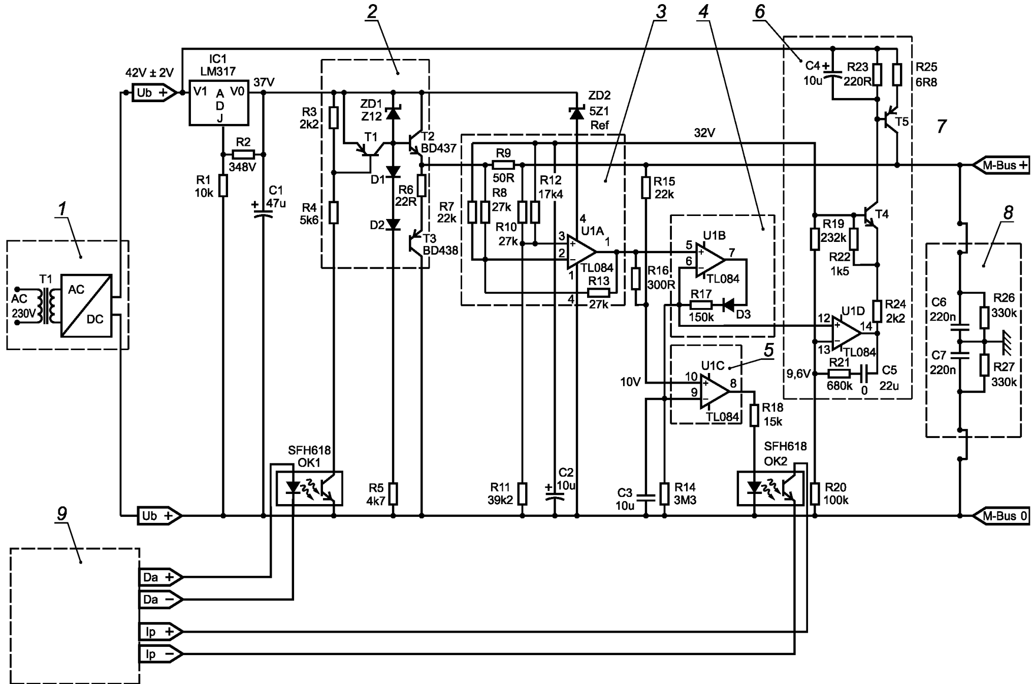
1 — источник питания с гальванической развязкой; 2 — программируемый источник напряжения; 3 — сдвиг уровня; 4 — детектор пикового напряжения; 5 — детектор сигнального напряжения; 6 — источник статического тока, макс. 400 мА; 7 — высокое усиление. Радиатор; 8 — симметричная сеть; 9 — защитное устройство управления
