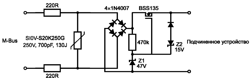
Рисунок Е.9 — Без заземления ( 100 \times 8 \text{ кВ} \times 1000 \text{ мкс} )
