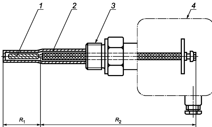
1 — термочувствительный элемент; 2 — защитный корпус; 3 — резьба для монтажа; 4 — соединительная головка; R_1 — сопротивление термочувствительного элемента; R_2 — сопротивление внутреннего провода и разъемов
