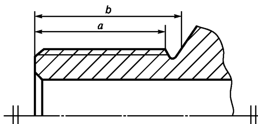
Рисунок 7 — Эскиз размеров a и b , указанных в таблице 4
