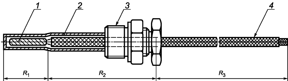
1 — термочувствительный элемент; 2 — защитный корпус; 3 — резьба для монтажа; 4 — кабель сигнала; R_1 — сопротивление термочувствительного элемента; R_2 — сопротивление внутреннего провода и разъемов; R_3 — сопротивление кабеля сигнала
