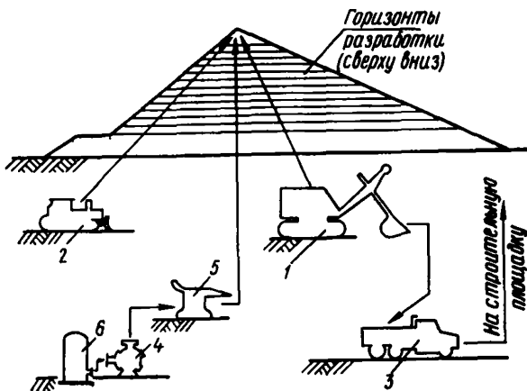
Рис. 6. Технологическая схема организации карьерных работ на терриконе
