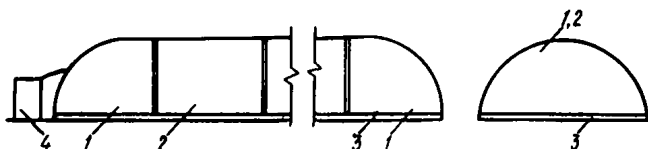
Рис. 9. Воздухоопорная оболочка
