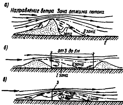
Рис. 13. Образование снежных отложений
