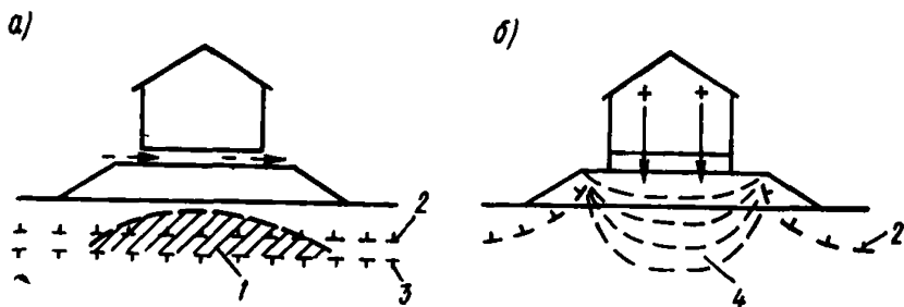
Рис. 7. Использование грунтов по I принципу (а) и по II принципу (б)
