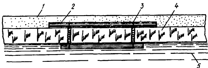
Рис. 18. Заделка сквозных трещин закреплением ледяных плит бревнами
