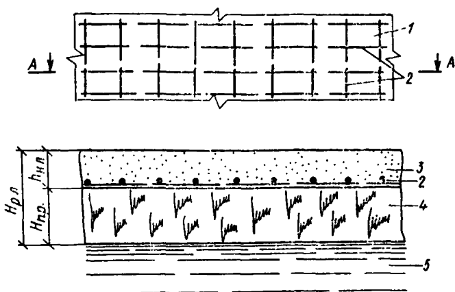
Рис. 19. Схема армирования ледяного покрова
