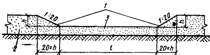
Рис. 12. Поперечный профиль летной полосы со снеговым покрытием 1 — переходные полосы (полосы сопряжения); 2 — снеговой покров; 3 — покрытие из уплотненного снега; l — ширина ГВП
