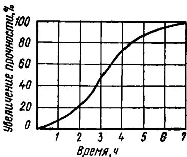
Рис. 10. График нарастания прочности уплотненного снега
