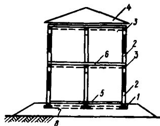
Рис. 5. Схема двухэтажного крупнопанельного здания на подсыпке
