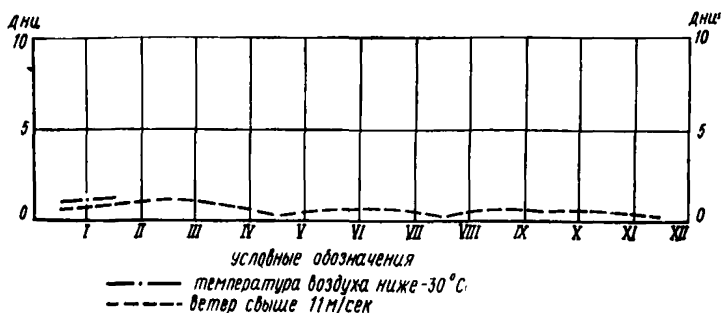
Рис. 1. График среднemesячной продолжительности воздействия природно-климатических факторов на производство III группы строительно-монтажных работ
