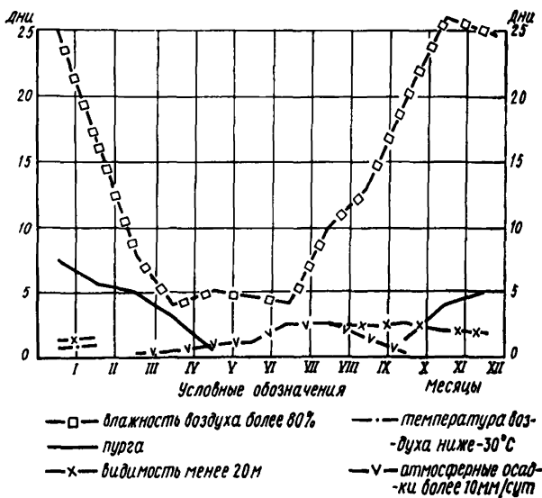
Рис. 4. График среднemesячной продолжительности воздействия природно-климатических факторов на производство II группы строительно-монтажных работ
