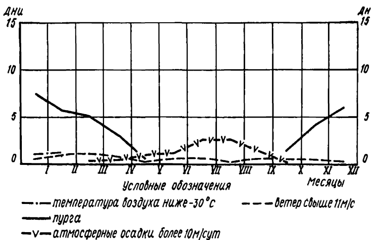
Рис. 2. График среднemesячной продолжительности воздействия природно-климатических факторов на производство IV группы строительно-монтажных работ
