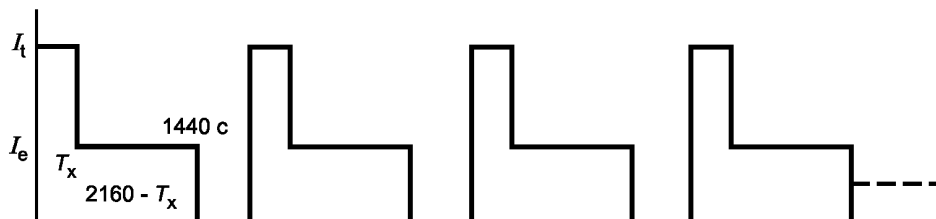
Профиль испытательного тока для AC-52a, AC-53a, AC-58a
