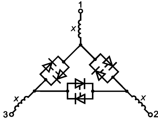
Рисунок 2б — Двигатель со схемой звезда, тиристоры со схемой треугольник;
