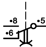
Переключающий контакт с замедлением в обоих направлениях
