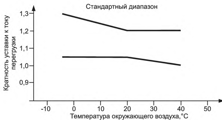
Рисунок 7 — Зависимости пределов кратности уставок тока от температуры окружающей воздуха для компенсированных реле перегрузки с выдержкой времени (см. 8.2.1.5.1)
