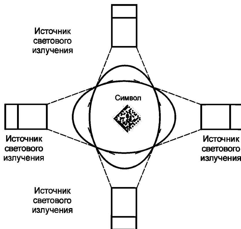
Рисунок 4 — Базовая оптическая схема (вид сверху)
