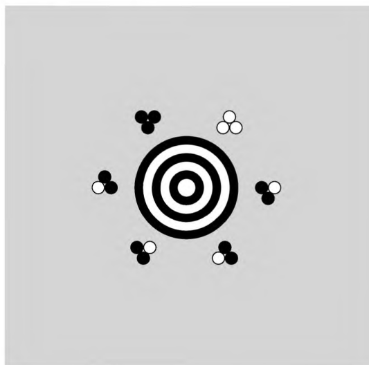
Рисунок А.1 — Фиксированные шаблоны в символе MaxiCode
