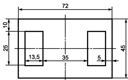
Рисунок Б.3 — Перегородка (вид сверху)
