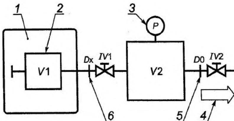
Рисунок G.1 - Схема испытания на неповреждаемость, описанного в 16.6.2 а)
