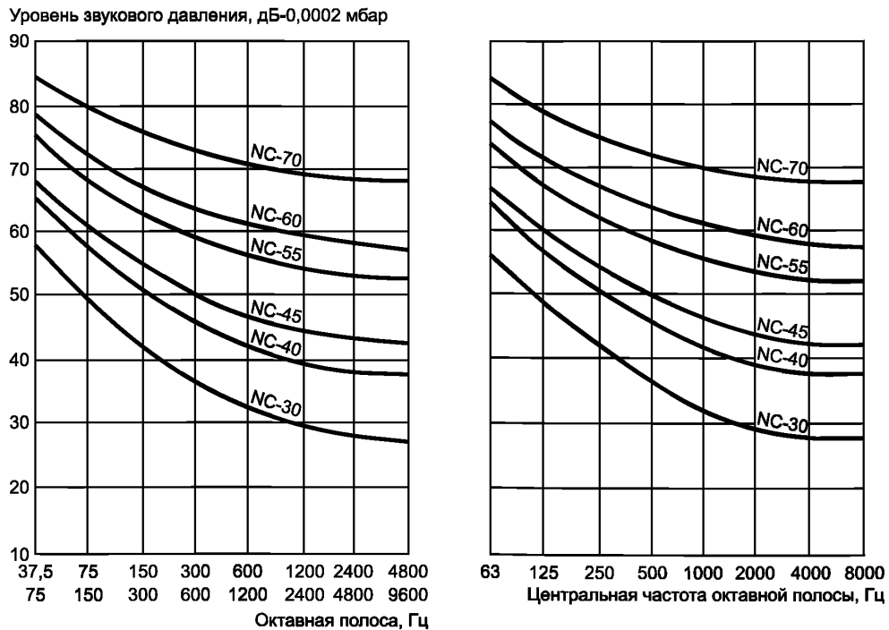
Рисунок 2 — Кривые зависимости критерия (NC) помех для телефонной связи
