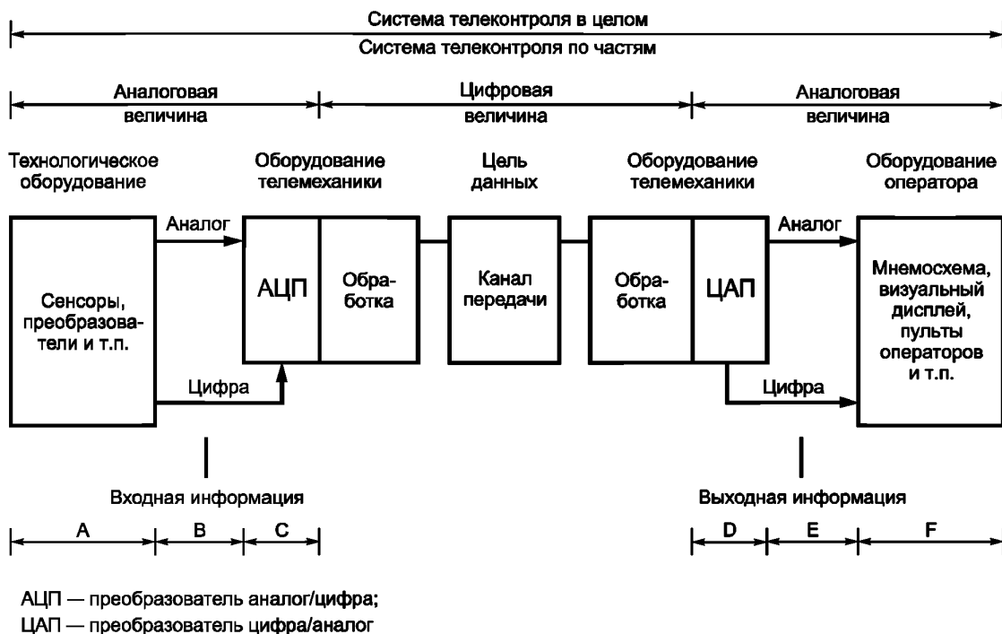
Рисунок 1 — Обработка аналоговой информации
