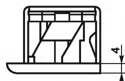
Рисунок Б.17 — Пример усиленной запорной планки коробчатой формы
