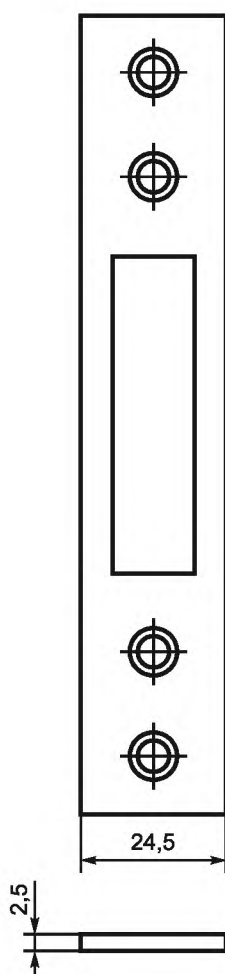
Рисунок Б.14 — Пример простой запорной планки
