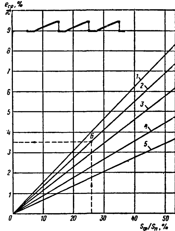
Рис. 12. График для определения среднего значения к. е. о. ( e_{ср} , %) в многопролетных производственных помещениях (три пролета и более) со светопроемами в плоскости покрытия (зевитными фонарями)
