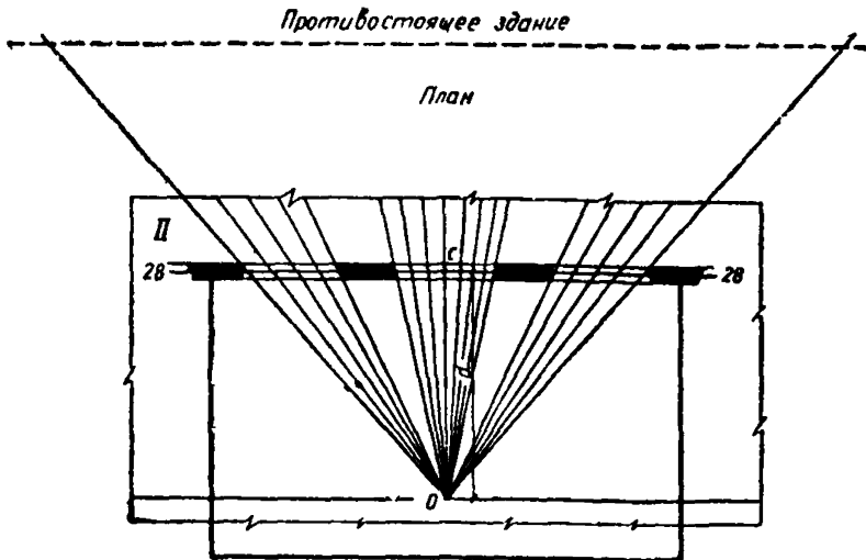
Рис. 27. Схема определения количества лучей на плане помещения
