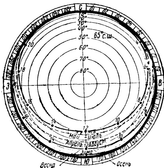
Рис. 40. Солнечная карта для расчета солнцезащитных средств в пределах расположения здания от 62,5 до 67,5° с. ш.
