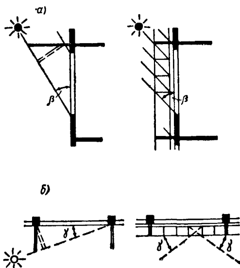
Рис. 2. Схема «защитных углов» козырьков, жалюзи и экранов
