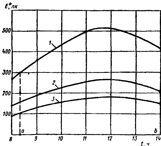
Рис. 34. График изменения естественной освещенности ( E^{\circ} , лк) в трех расчетных точках школьного класса в течение рабочего дня
