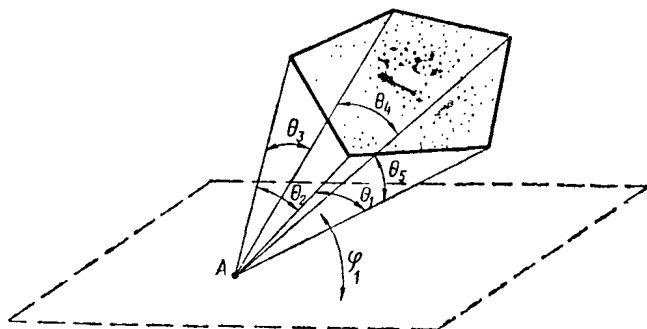
Рис. 22. Схема для определения к. е. о. от светового проема, имеющего форму многоугольника
