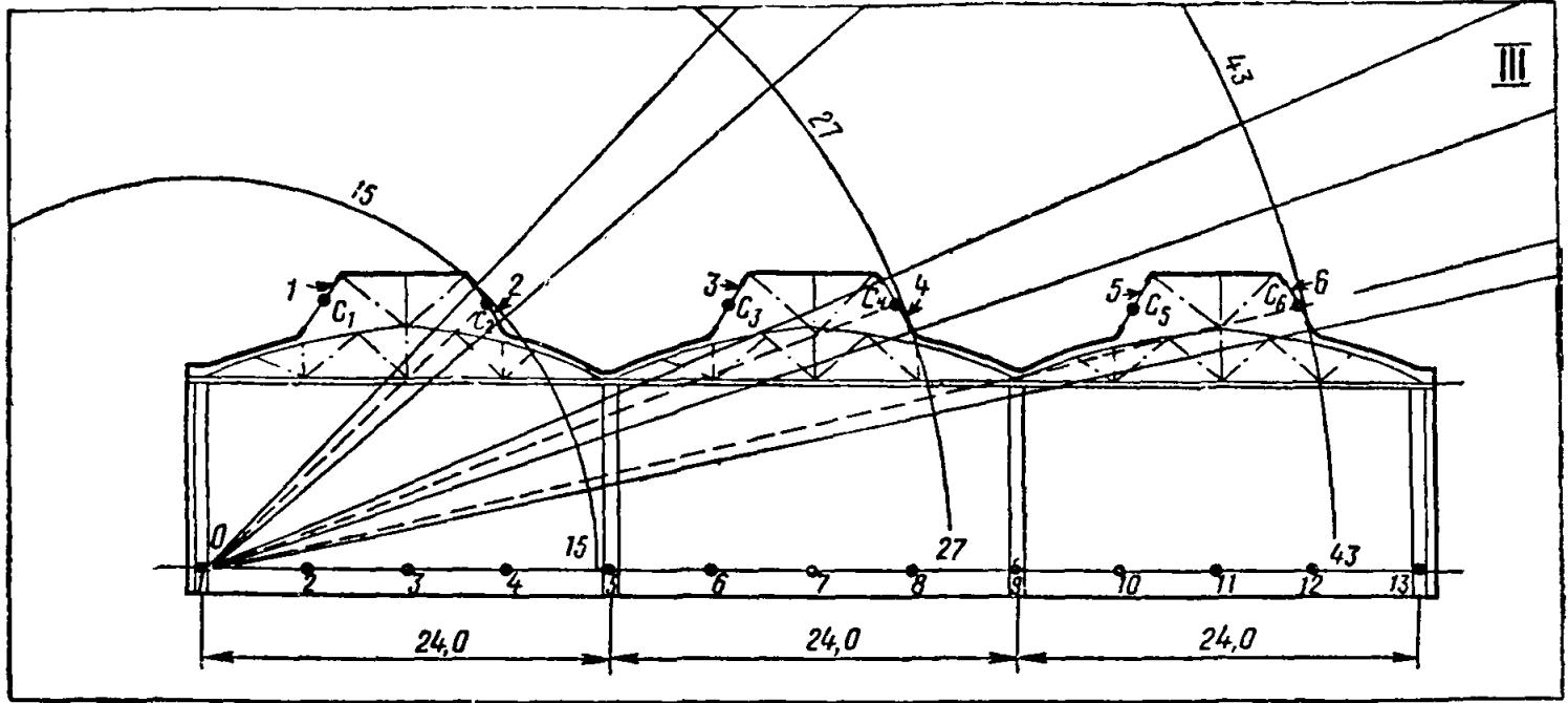
Рис. 29. Схема трехпролетного производственного помещения с трапециевидными фонарями
