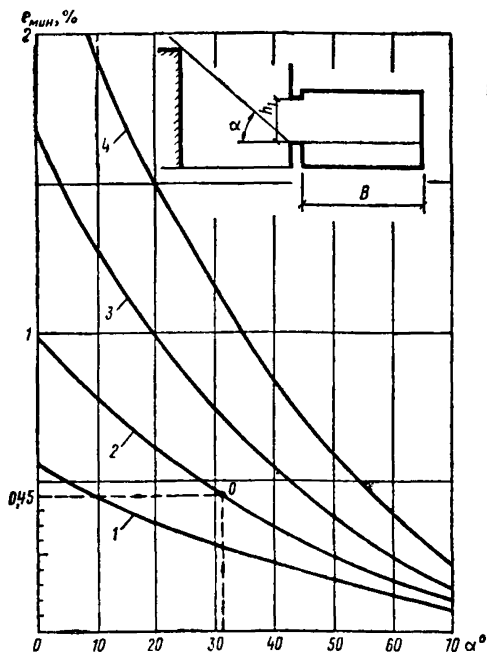
Рис. 7. Зависимость минимального значения к. е. о. ( \epsilon_{\min} , %) в жилых помещениях от глубины помещения B и угла затенения окна противостоящим зданием протяженного типа
