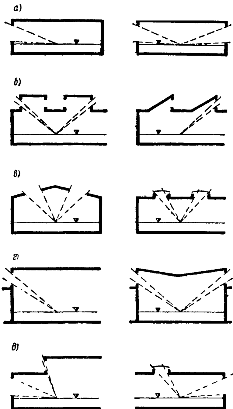
Рис. 1. Схемы естественного освещения зданий
