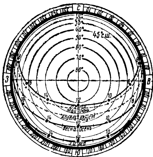
Рис. 38. Солнечная карта для расчета солнцезащитных средств в пределах расположения здания от 42,5 до 47,5° с. ш.
