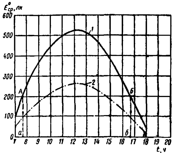
Рис. 32. График изменения естественной освещенности в помещении в течение рабочего дня
