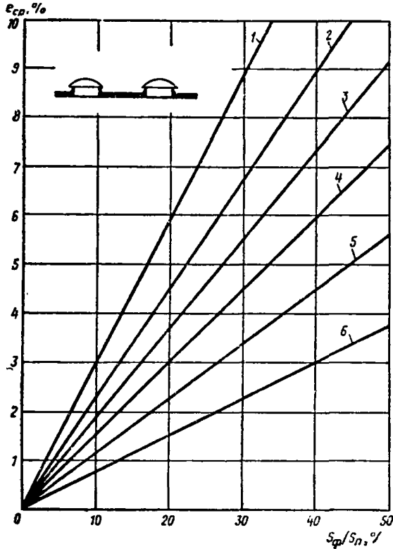
Рис. 12. График для определения среднего значения к. е. о. ( e_{ср} , %) в многопролетных производственных помещениях (три пролета и более) со светопроемами в плоскости покрытия (зевитными фонарями)
