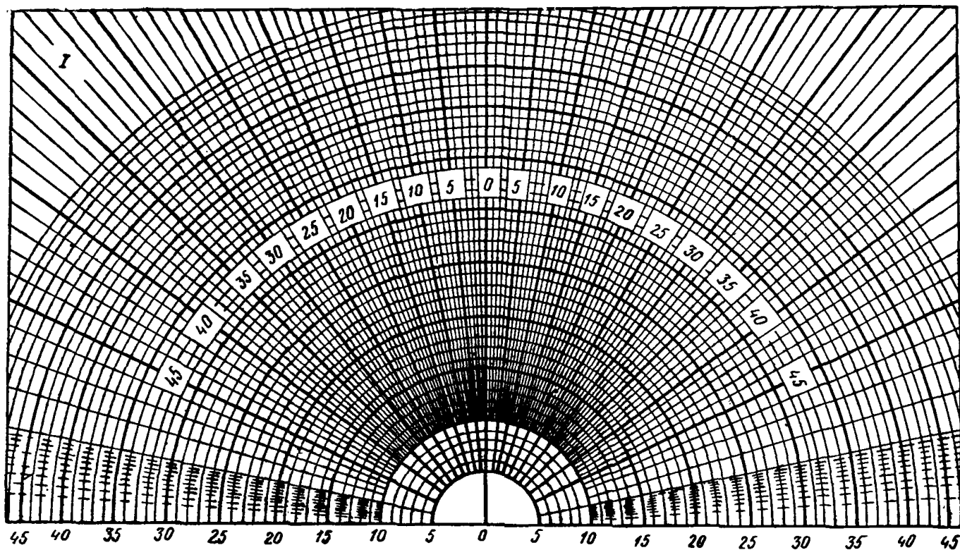
Рис. 15. График 1 для подсчета количества лучей n_1 и n_1' , проходящих через световой проем на характерном поперечном разрезе помещения при боковом освещении (цифры на полуокружности обозначают количество лучей, на нижней горизонтальной линии — номера полуокружностей)
