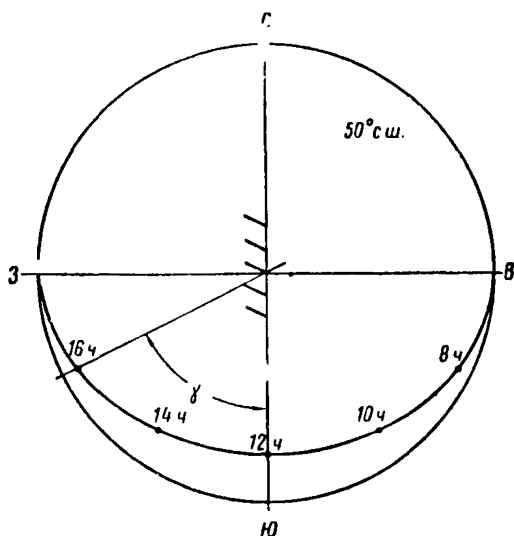
Рис. 41. Схема расположения вертикальных экранов в плане, \gamma — «защитный угол» вертикальных экранов
