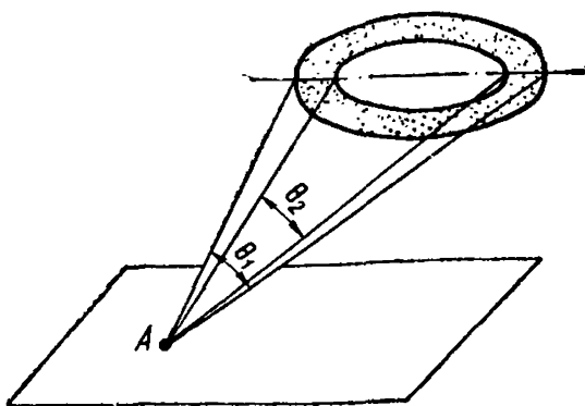
Рис. 21. Схема для опреде- ления к. е. о. от светопроема кольцеобразной формы в по- крытии
