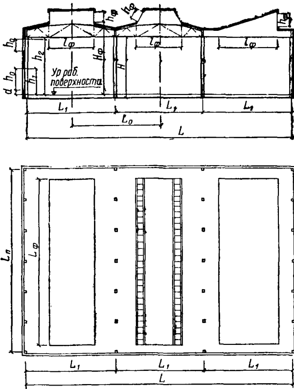
Рис. 9. Условные обозначения основных размеров помещений и световых проемов при верхнем и комбинированном естественном освещении
