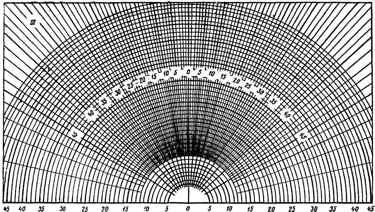
Рис. 18. График III для подсчета количества лучей n_3 , проходящих через световые проемы на поперечном разрезе помещения при верхнем освещении (цифры на полуокружности обозначают количество лучей, на нижней горизонтальной линии — номера полуокружностей)
