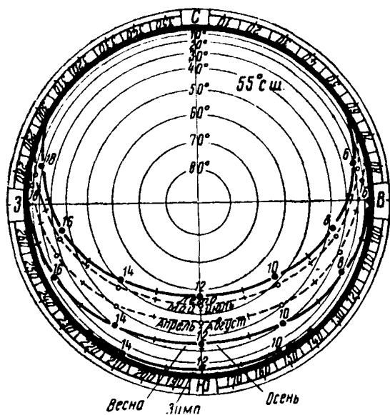
Рис. 39. Солнечная карта для расчета солнцезащитных средств в пределах расположения здания от 52,5 до 57,5° с. ш.
