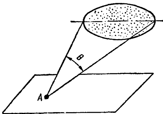
Рис. 20. Схема для опреде- ления к. е. о. от светопро- емов круглой формы в по- крытии
