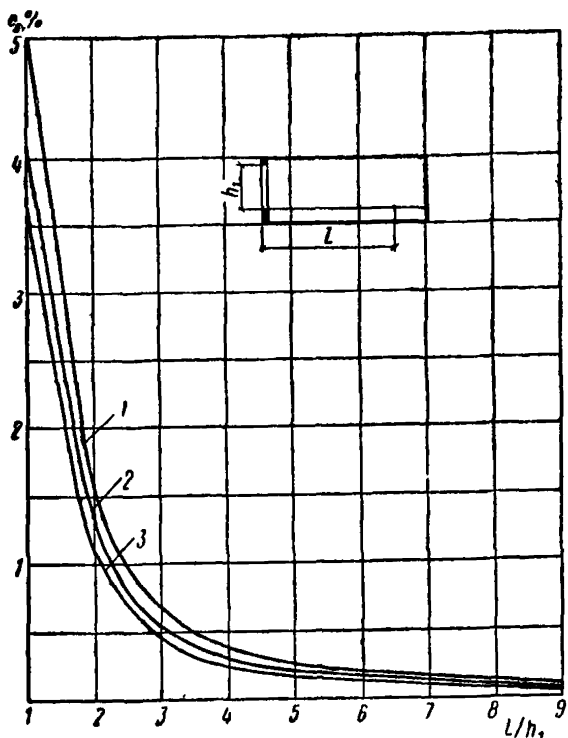
Рис. 5. Зависимость к. е. о. ( e , %) в точках характерного разреза помещения от отношения l/h_1 и типа заполнения отдельных окон
