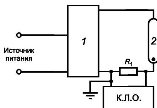
1 — испытуемый ПРА; 2 — номинальная лампа; К.Л.О. — осциллограф
