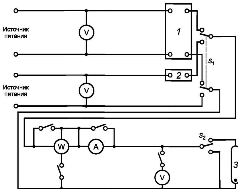
1 — испытуемый ПРА; 2 — ДОО; 3 — номинальная лампа
