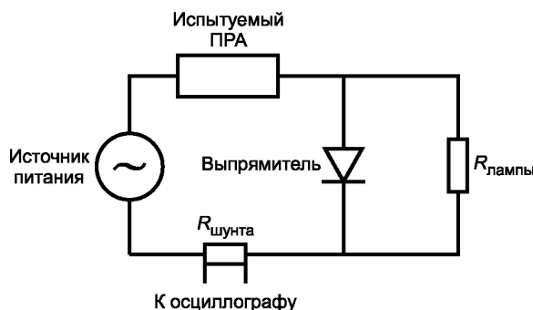
Рисунок 3 — Схема испытания пускового тока лампы
