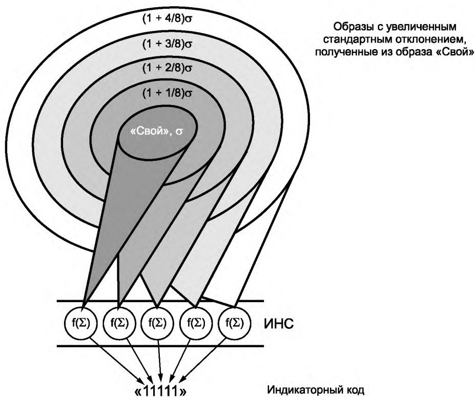
Рисунок Г.1 — Обучение ИНС мягкого индикатора на образцах с возрастающим среднеквадратичным отклонением
