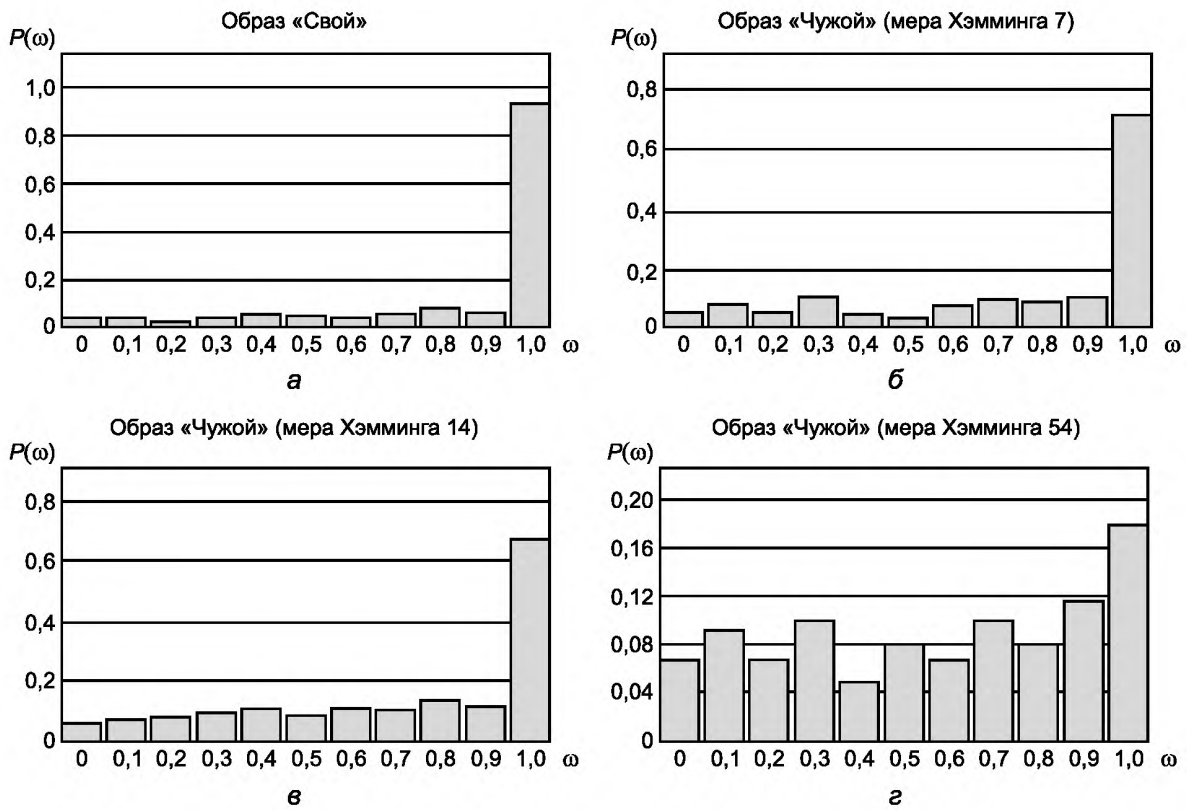
Рисунок Б.1 — Распределения показателей стабильности примеров образа «Свой» и образов «Чужой» для выходного кода длиной 256 разрядов, отличающихся от образа «Свой» по мере Хэмминга:
