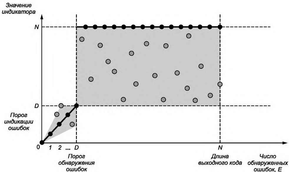
Рисунок 3 — Функция значений мягкого индикатора
