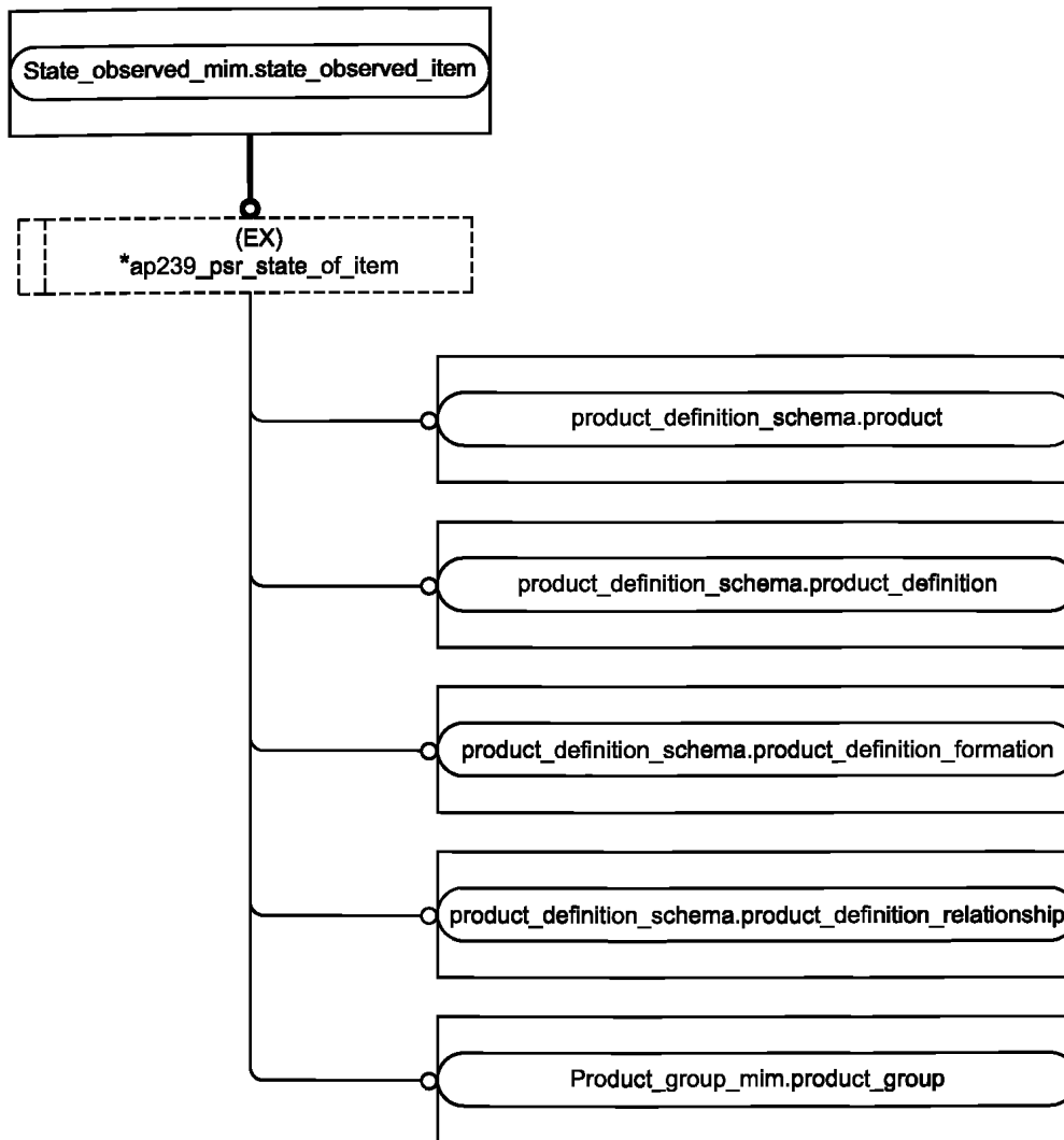
Рисунок D.2 — Представление ИММ на уровне объектов в формате EXPRESS-G (диаграмма 1 из 4)
