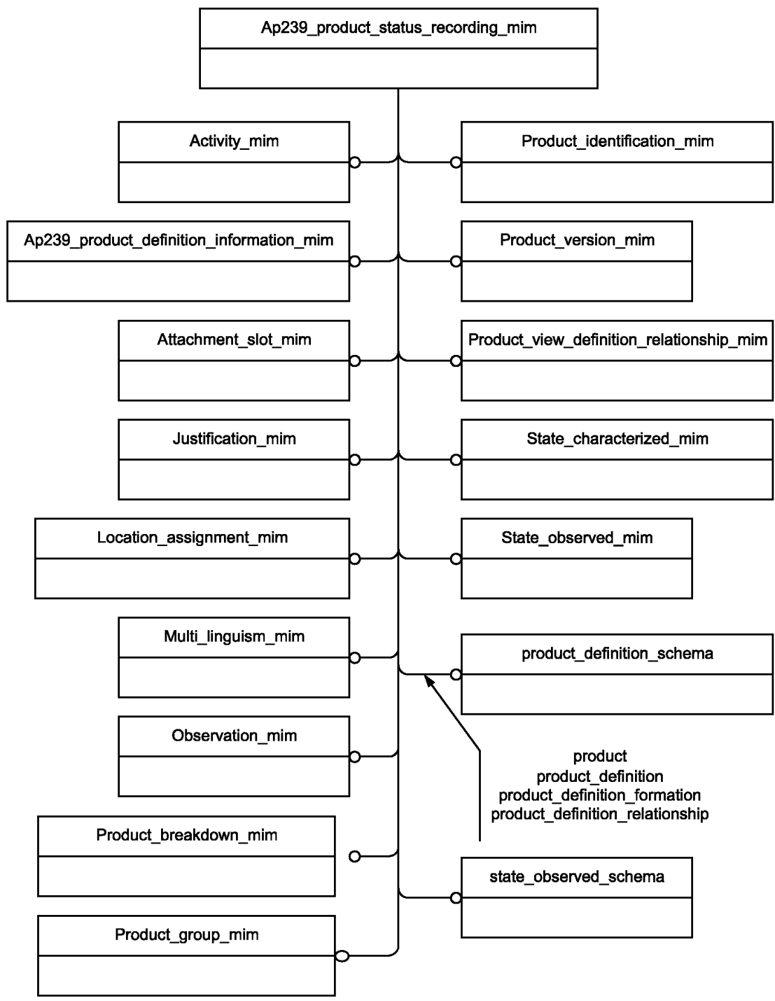
Рисунок D.1 — Представление ИММ на уровне схем в формате EXPRESS-G (диаграмма 1 из 1)
