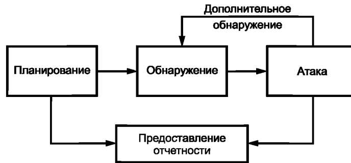
Рисунок 1 — Методика испытаний четырехэтапного проникновения в сеть
