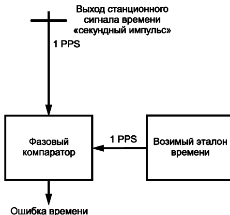
Рисунок 4 — Контроль качества временной синхронизации
