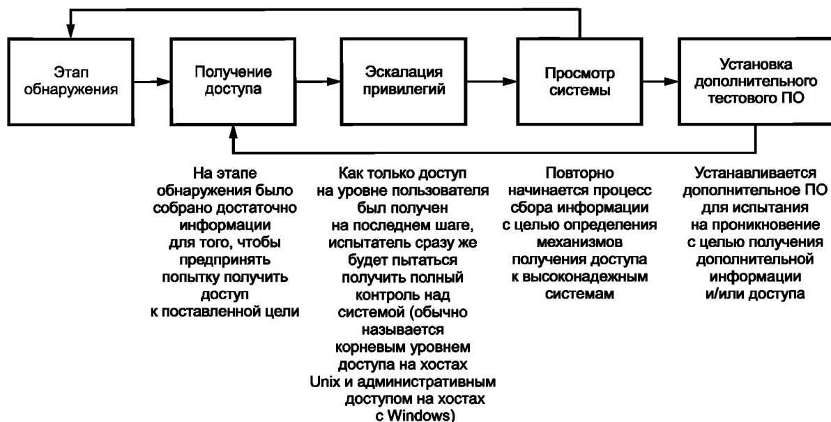
Рисунок 2 — Этапы атаки с петлей обратной связи
