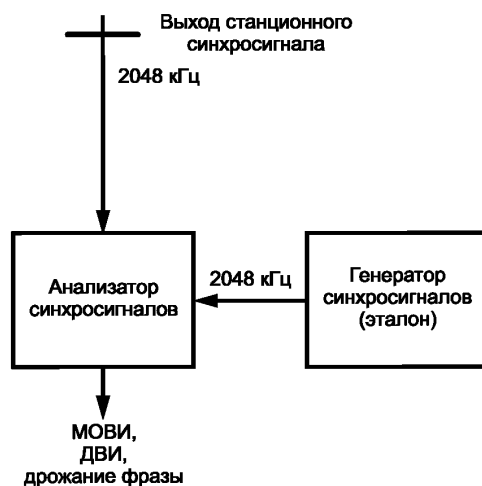
Рисунок 3 — Контроль качества частотной синхронизации
