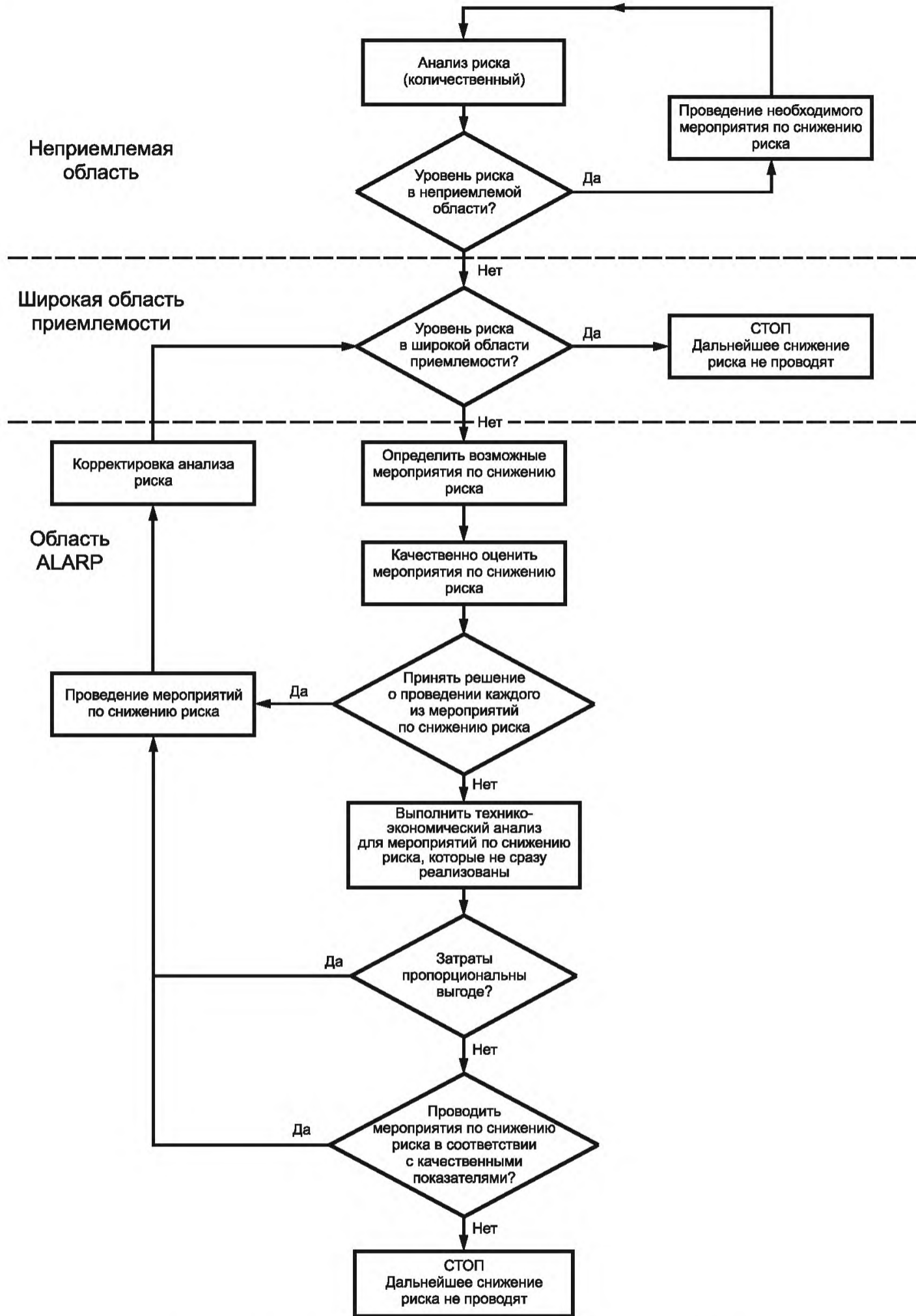
Рисунок Г.2 — Демонстрация использования принципа ALARP
