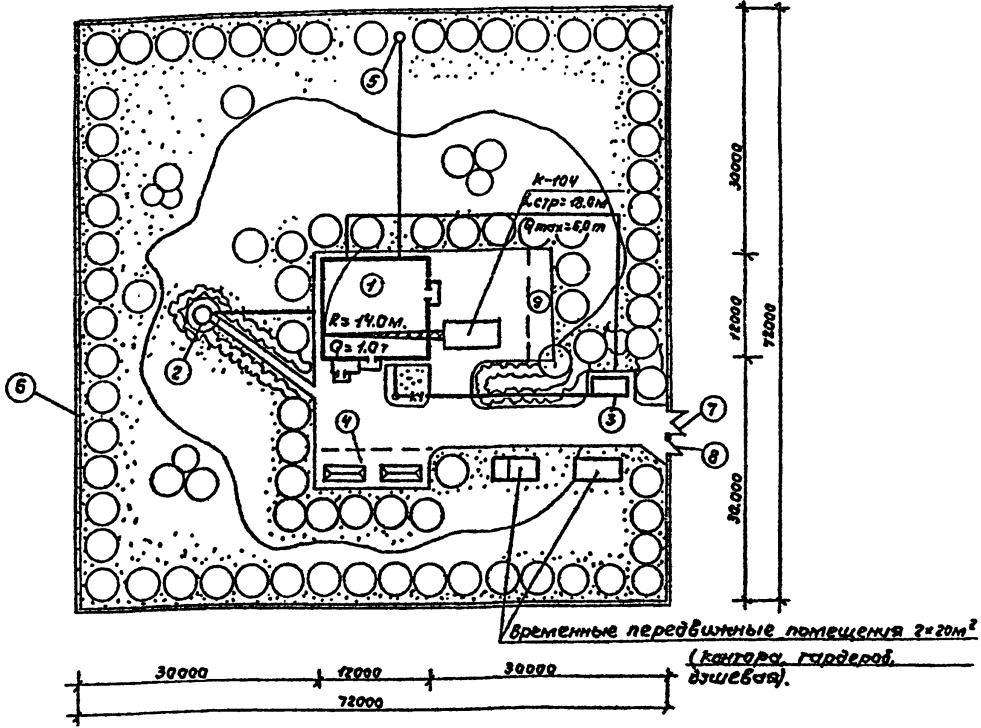
Схема генплана Q=800 м³/сут.
