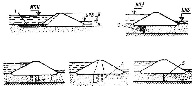
Рис. 2. Конструкции противофильтрационных устройств в основании 1 — понур; 2 — зуб; 3 — инъекционная завеса; 4 — то же, высячая; 5 — диафрагма (стенка, шпунт)
