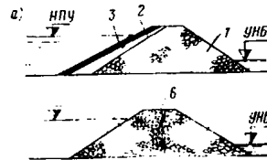
Рис. 8. Виды каменнонабросных плотин
