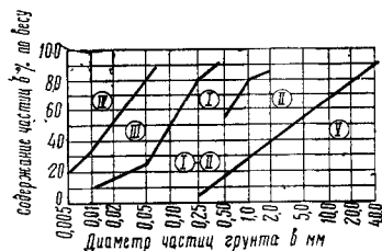
Рис. 6. Группы грунтов, используемых для намыва плотин
