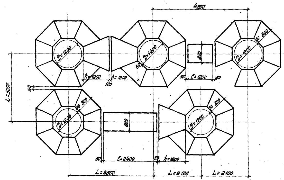
Схема 13
