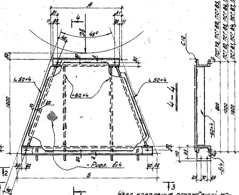
Узел крепления ограждений марок ПЛ 26, ПЛ 27, ПЛ 28 в торцах ограждений
