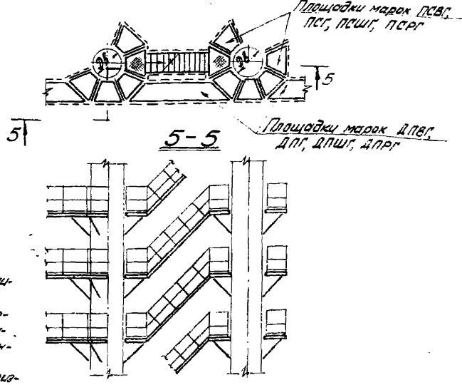
Схема лестницы №5
