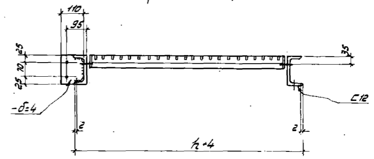
1-1 (повернута)
