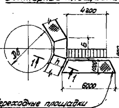
Секторные площадки
