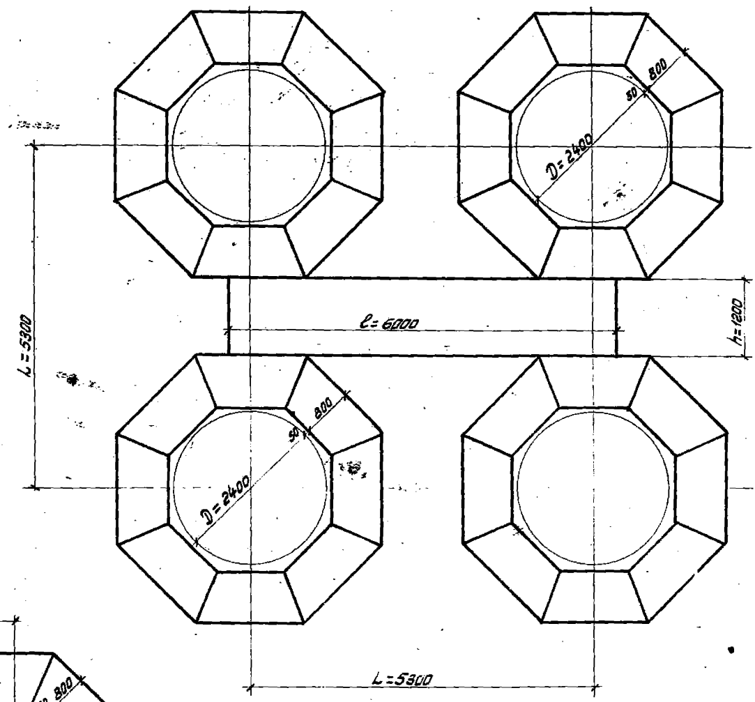
Схема 12
