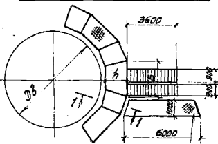
Комбинированные площадки
