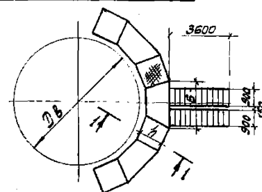
Комбинированные площадки
