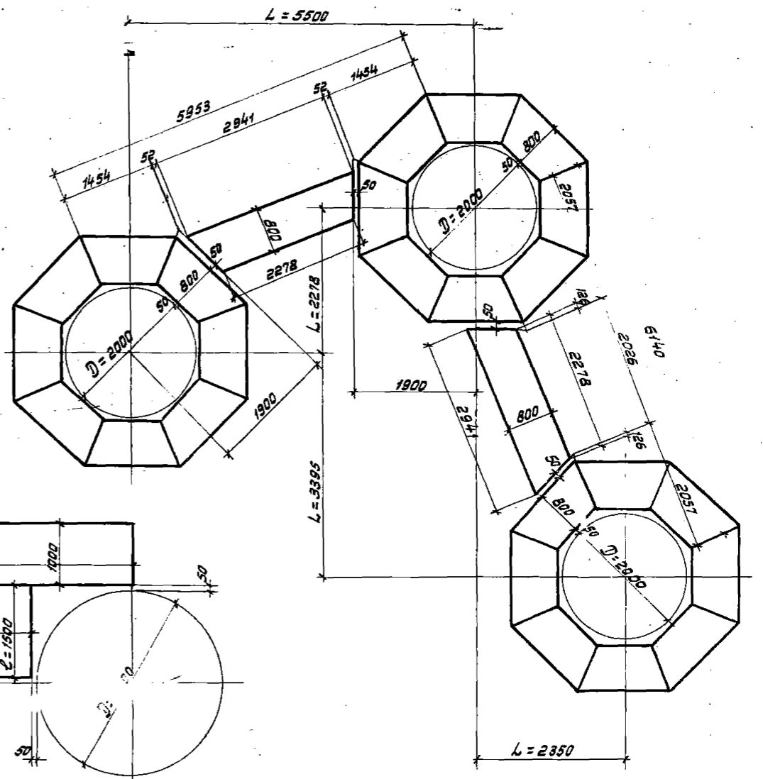
Схема 15
