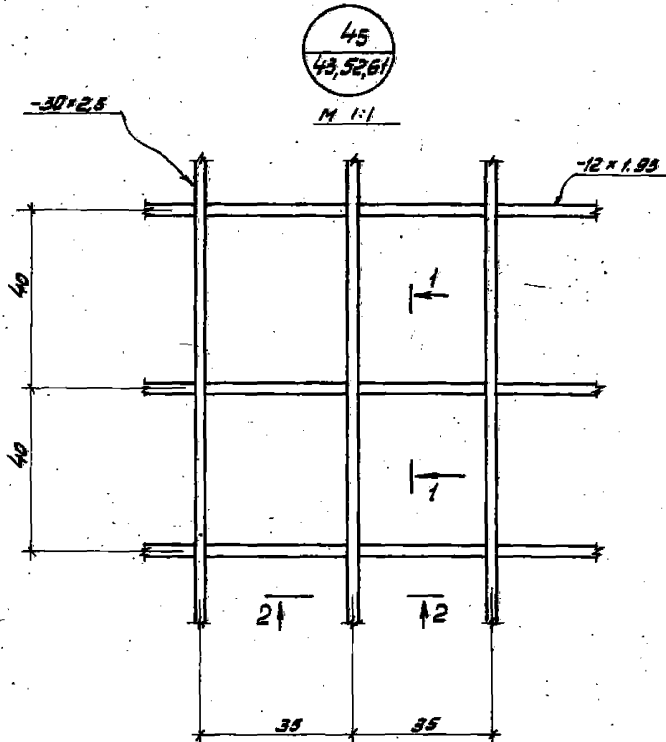
Детали вырезов в планках -30 \times 2.5 , -12 \times 1.95
