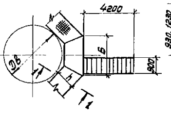
Секторные площадки
