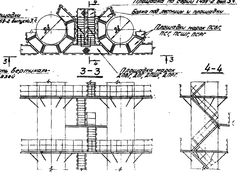
Схема лестницы №5
