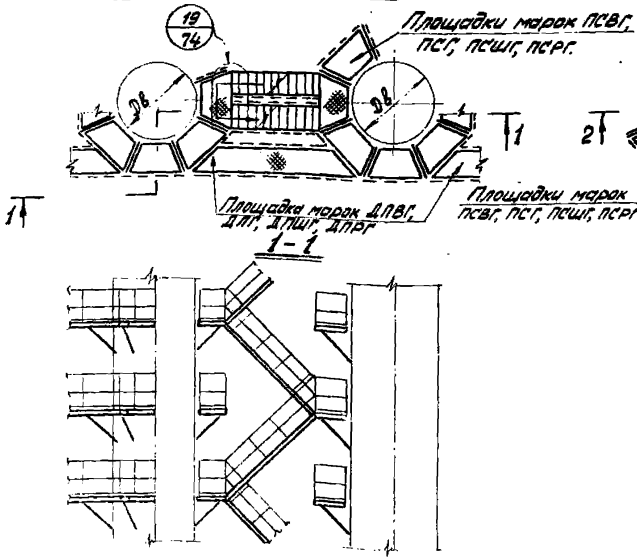
Схема №4 лестницы и площадки
