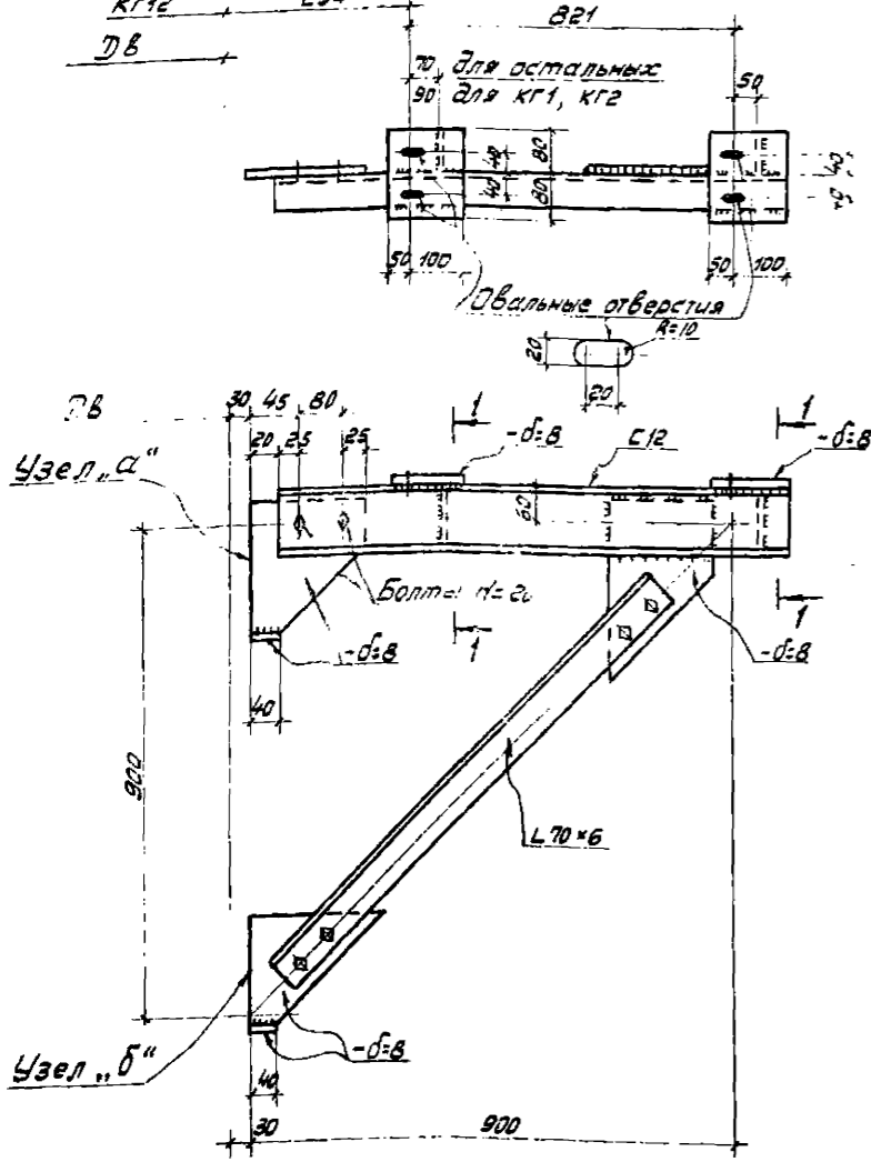
Узел „а“
