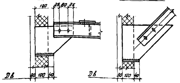
Узел „а“
