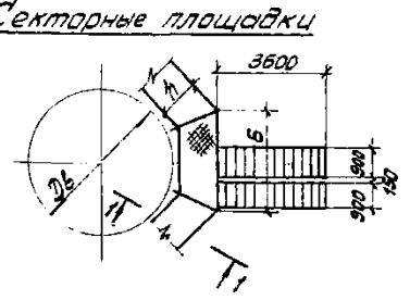
Секторные площадки
