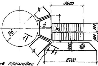
Секторные площадки
