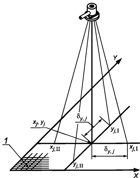
1 — пластинка с сеткой штрихов x-y
