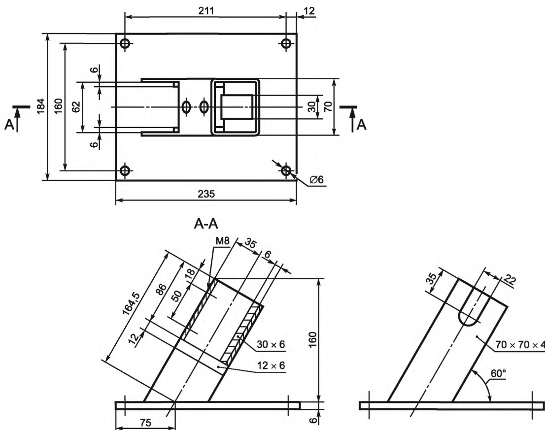
Рисунок 3 — Опорный стенд
