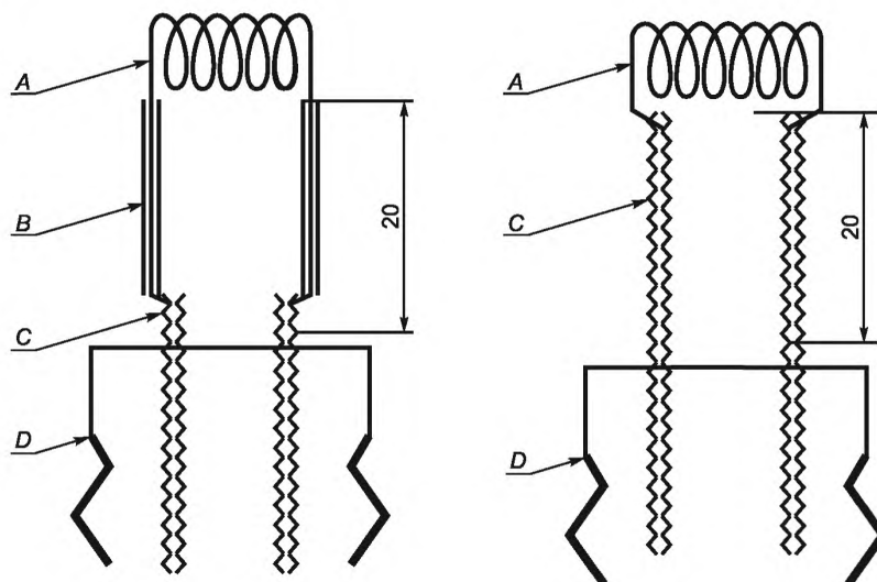
А — катушка зажигания; В — изоляция; С — электроды; D — запальная пробка
