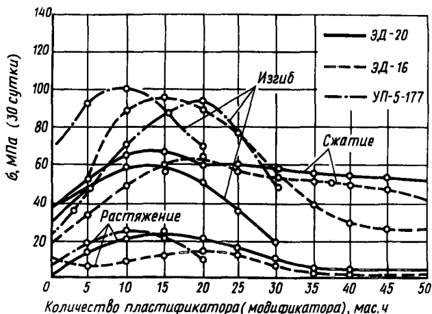
Рис. 47. График подбора состава ЭКП в зависимости от когезионной прочности при изменении количества пластификатора
