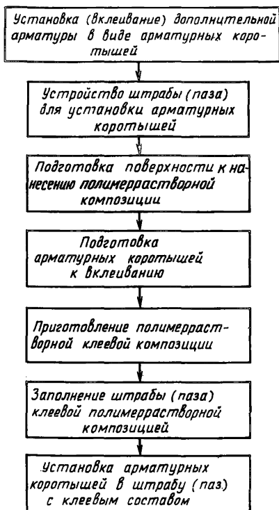
Рис. 54. Пооперационная технологическая схема установки коротышей
