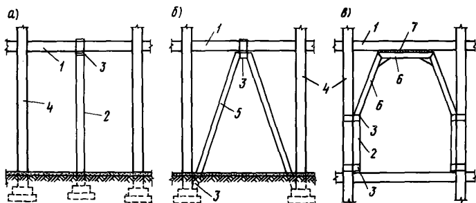
Рис. 37. Конструкции частичного разгружения
