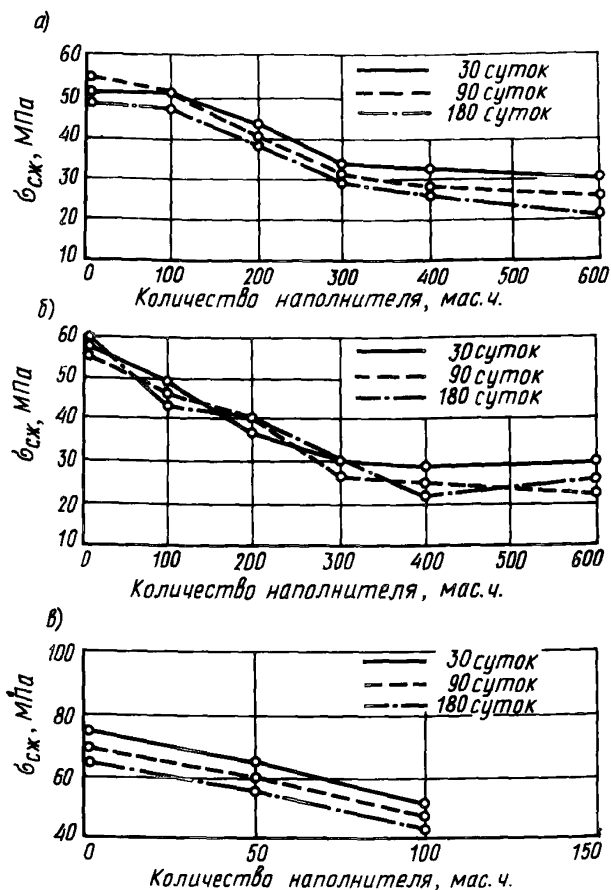
Рис. 51. Атмосферостойкость полимеррастворов в зависимости от количества наполнителя (ПК) а – смола ЭД-20; б – смола ЭД-16; в – смола УП-5-177
