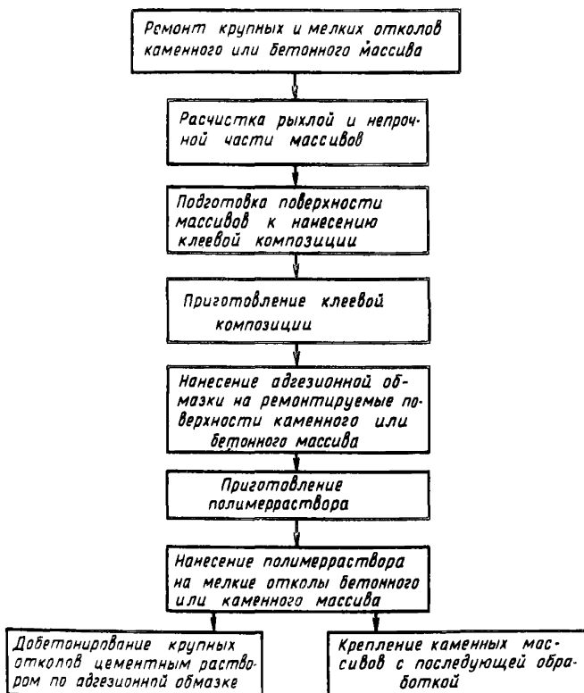
Рис. 53. Схема операций при ремонте отколов
