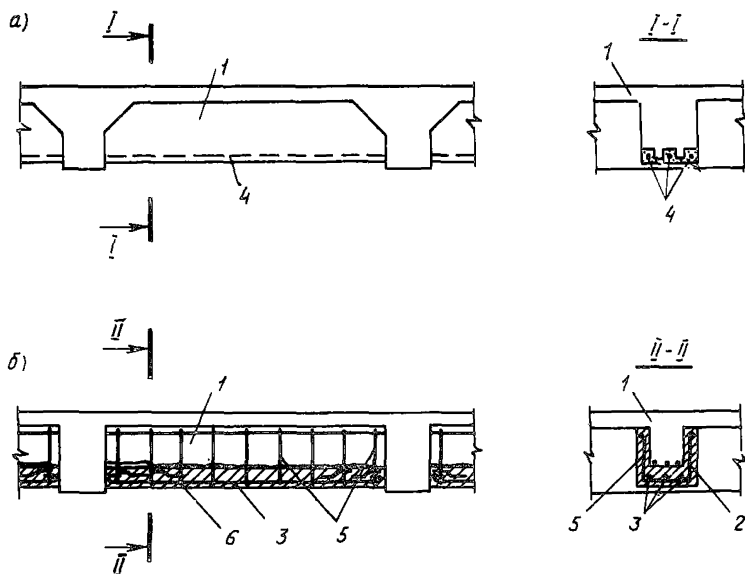
Рис. 40. Усиление изгибаемых конструкций
