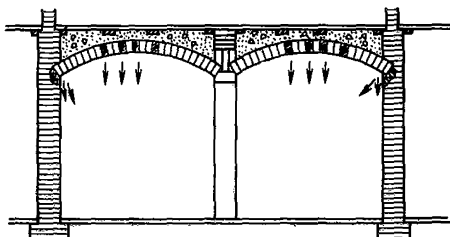
Рис.14. Характерные повреждения в плоском цилиндрическом сводчатом перекрытии (помещение разделено подпружной аркой на две части)
