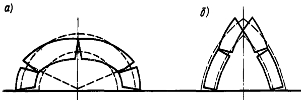
Рис.22. Схема разрушения арок под вертикальными нагрузками
