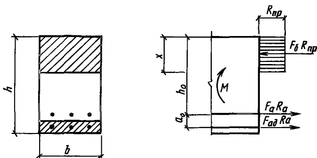
Рис.44. Расчетная схема балки при усилении обоймой, рубашкой, наращиванием
