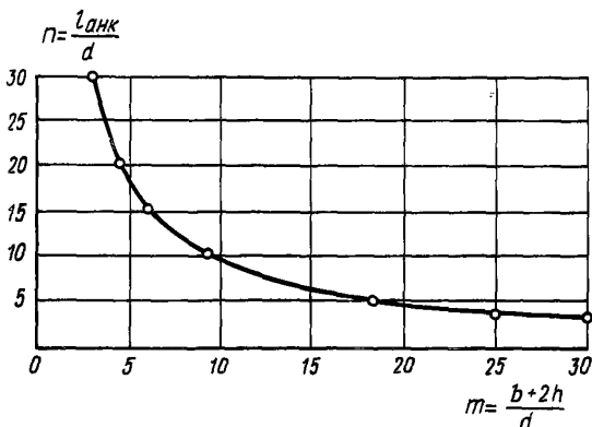
Рис. 45. График выбора периметра бетонной штрабы в зависимости от длины заделки арматурного стержня
