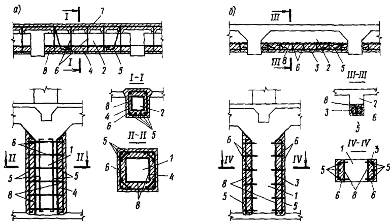
Рис. 39. Усиление сжатых и изгибаемых конструкций а – железобетонными обоймами; б – наращиванием бетона; 1 – усиливаемая колонна; 2 – усиливаемая балка; 3 – конструкция наращивания; 4 – обойма; 5 – стержни усиления; 6 – хомуты; 7 – отверстие для установки хомутов и подачи бетона; 8 – адгезионная обмазка полимерным раствором по обработанной поверхности конструкции
