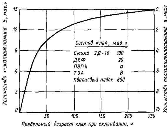
Рис. 69. График для подбора рецептуры ЗКП с комбинированным отвердителем при температуре 20–50°C, обеспечивающая \sigma от 50 кгс/см 2
