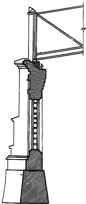
Рис.17. Характерные повреждения при опирании большепролетной металлической конструкции на контрфорсе
