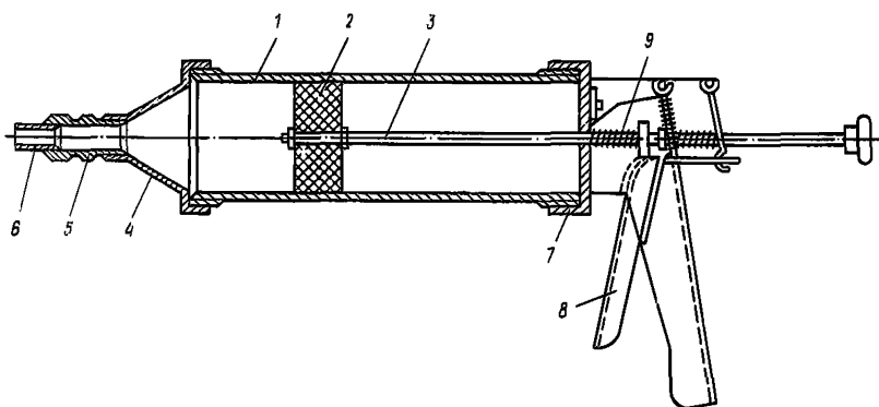
Рис. 58. Механический пистолет для нанесения и инъектирования полимерраствора в трещины
