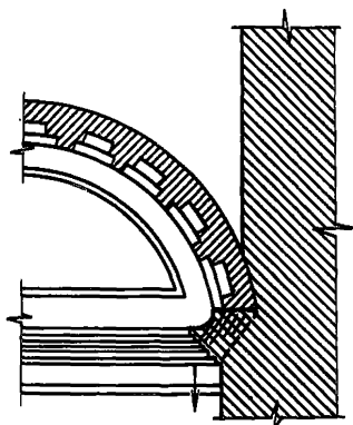
Рис.15. Повреждения в конструкции кессона в цилиндрическом своде
