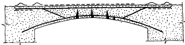
Рис.29. Трещины в своде с горизонтальной верхней поверхностью, проскальзывание верхней арматуры и коррозия плиты
