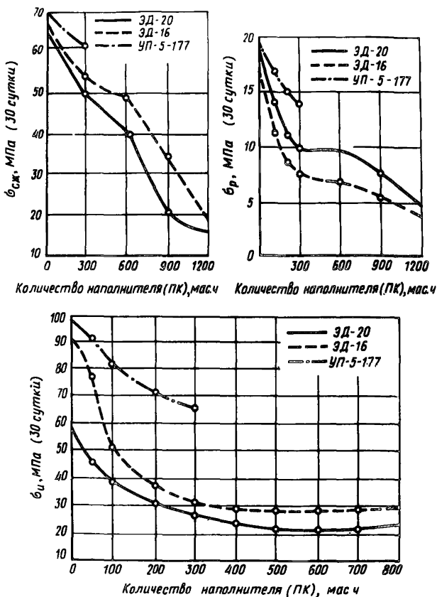
Рис.49. График подбора состава ЗКП в зависимости от когезионной прочности при изменении количества наполнителя
