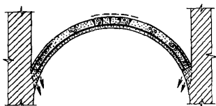
Рис. 24. Трещины в железобетонной потолочной плите, коррозия нижних полок металлических балок и выпучивание бетона
