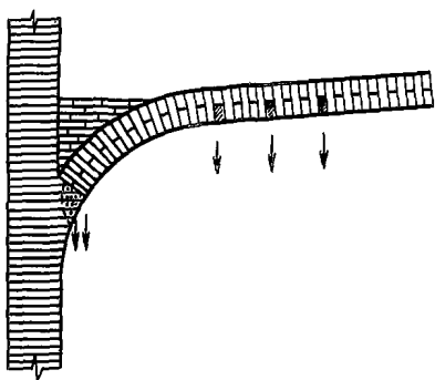
Рис.9. Повреждения в зеркальном своде с пятами подлуг, образованными выпускными рядами кладки опорных стен
