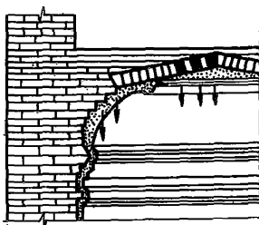
Рис.13. Повреждения в зеркальном своде (с поддугами в виде выпуклых рядов)
