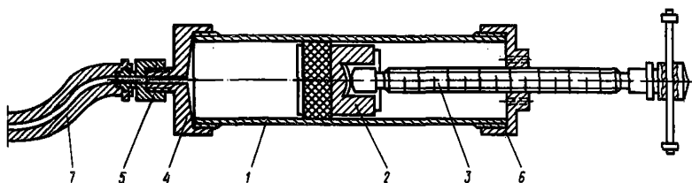
Рис. 56. Шприц-инъектор ОИСИ для нагнетания полимерраствора в трещины
