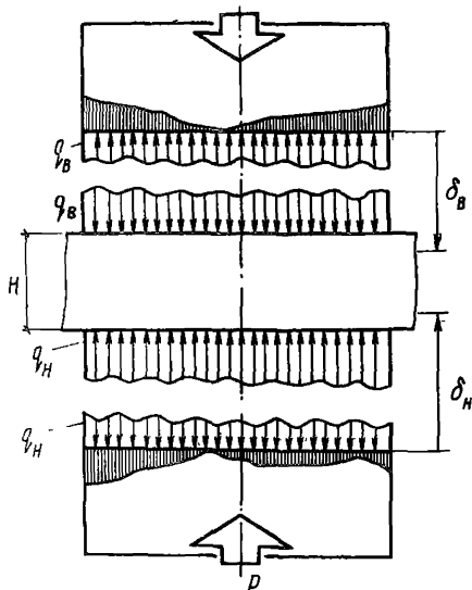
Рис. 62. Клеевая прокладка между массивами с неровными поверхностями контакта
