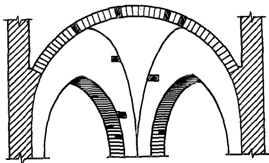
Рис.7. Повреждения в парусно-сомкнутом своде
