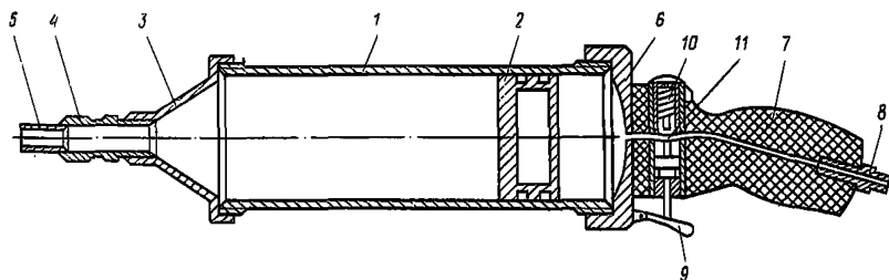
Рис. 57. Пневматический пистолет для нанесения и инъектирования полимерраствора
