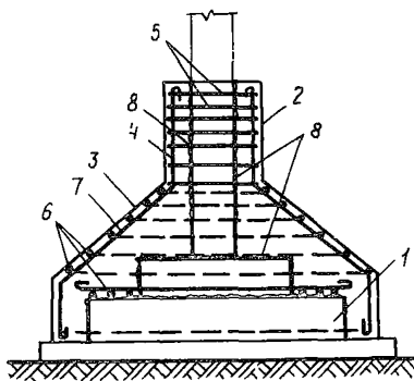
Рис. 41. Усиление фундамента железобетонной рубашкой
