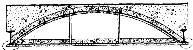
Рис.28. Трещины и коррозия нижней полки двутавра в сводчатом потолке с подвешенной плоской плитой
