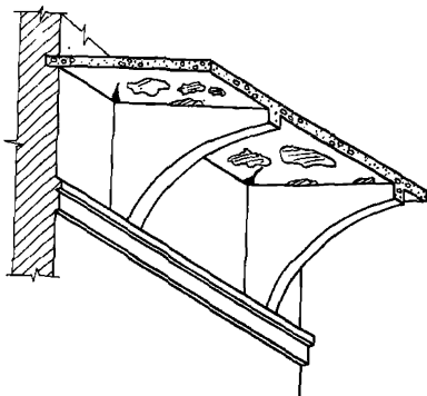
Рис.27. Повреждения в ребристом своде (покрытие между ребрами плоского вида)
