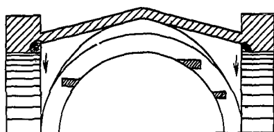
Рис.8. Повреждения в конструкции впаушенного крестового свода
