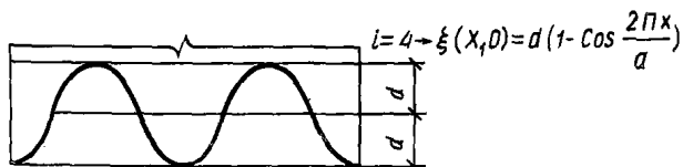
Рис. 65. Характеристика поверхности "гармонические неровности"
