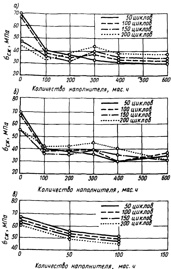
Рис.50. Морозостойкость полимеррастворов в зависимости от количества наполнителя (ПК) а – смола ЭД-20; б – смола ЭД-16; в – смола УП-5-177
