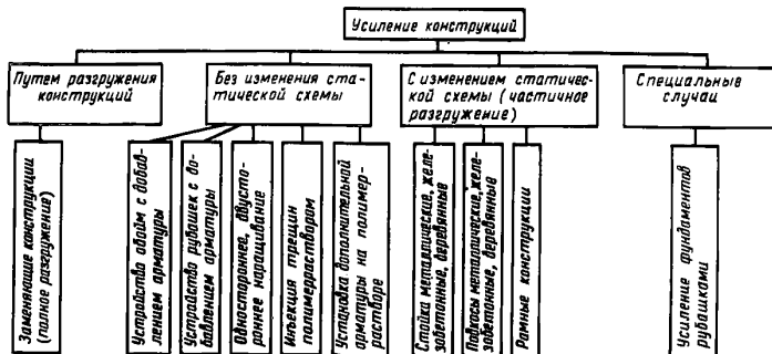
Рис.36. Классификация способов усиления конструкций зданий и сооружений при проведении реставрационных работ
