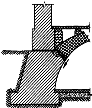
Рис.18. Трещины в пяте свода, опирающегося на фундамент
