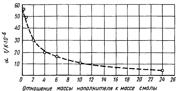
Рис. 48. График подбора состава ЭКП в зависимости от коэффициента линейного расширения
