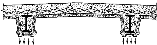
Рис. 23. Повреждения в металобетонном перекрытии (коррозия нижней полки двутавра)
