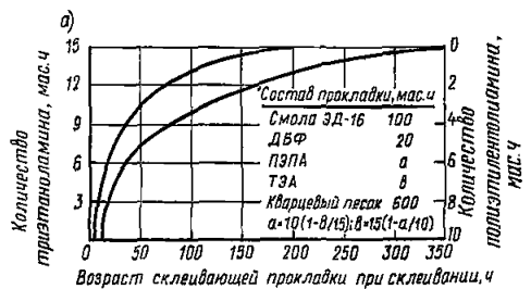
Рис. 69. График для подбора рецептуры ЗКП с комбинированным отвердителем при температуре 20–50°C, обеспечивающая \sigma от 50 кгс/см 2
