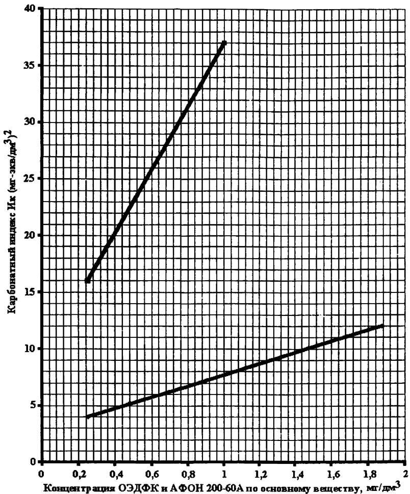
Рис.2 Область применения ОЗДФК, АФОН 200-60А и их аналогов, проверенных и сертифицированных в РАО «ЕЭС России», для систем теплоснабжения и ГВС при температуре не более 100 0 С и нагреве в водогрейных водотрубных котлах
