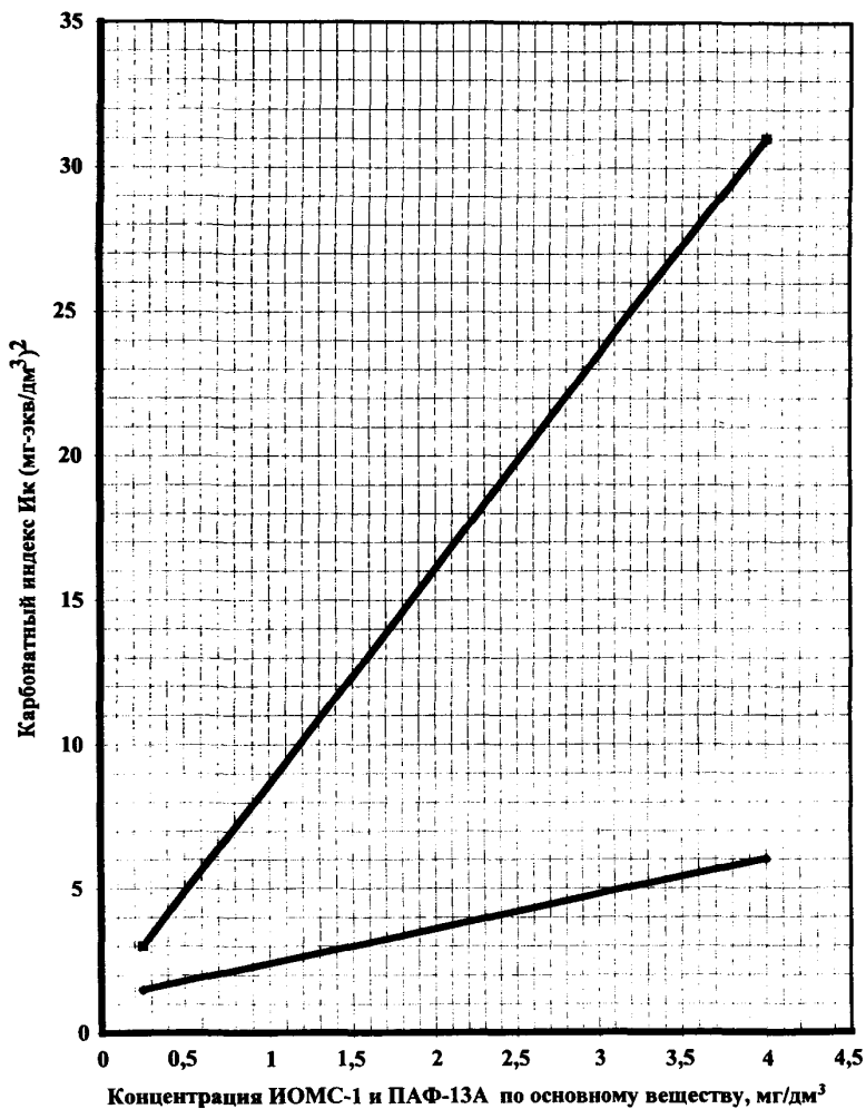
Рис.6 Область применения ИОМС-1, ПАФ-13А и их аналогов, проверенных и сертифицированных в РАО «ЕЭС России», для систем теплоснабжения при температуре 101-135 0 С и нагреве в водогрейных водотрубных котлах.
