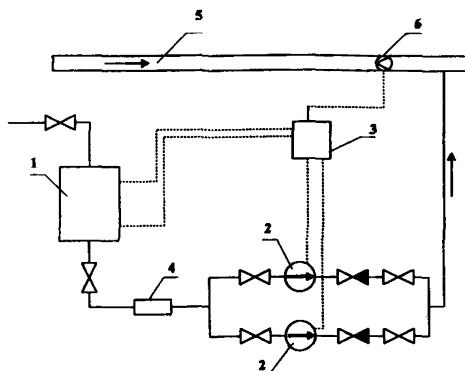
1 – расходный бак раствора реагента; 2 – насос-дозатор; 3 – блок управления; 4 – фильтр; 5 – стационарный трубопровод; 6 – расходомер.
