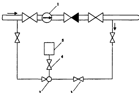
1 – штатный насос; 2 – эжектор; 3 – регулирующий клапан; 4 – регулирующий клапан; 5 – расходный бак раствора реагента.
