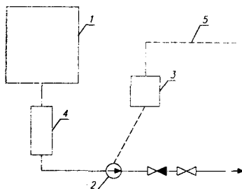
1 – расходный бак раствора реагента; 2 – насос; 3 – блок управления; 4 – фильтр; 5 – сигнал от штатных насосов.
