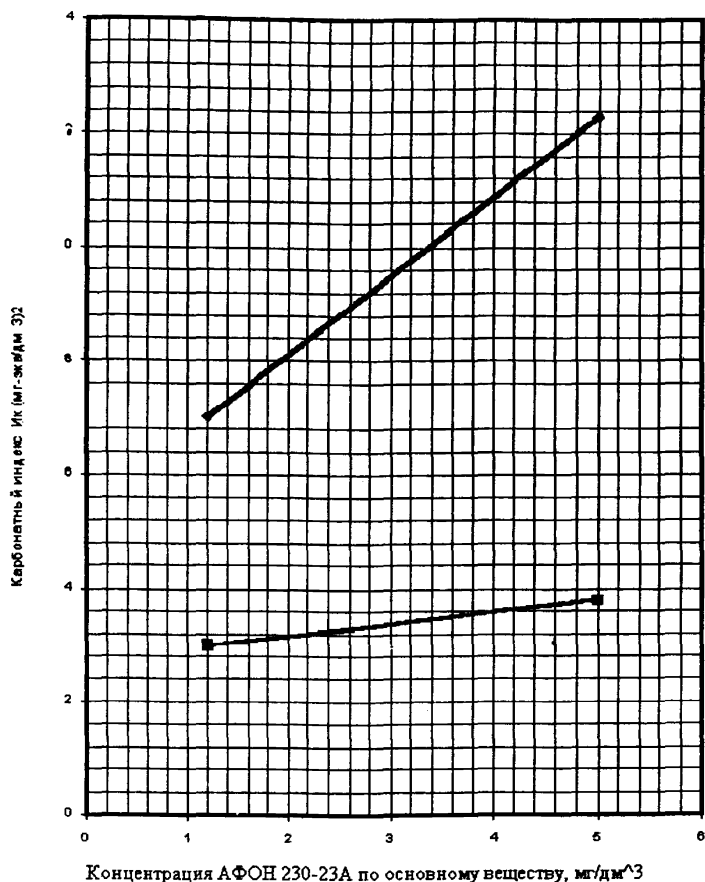
Рис.7. Область применения АФОН 230-23А и его аналогов проверенных и сертифицированных в РАО «ЕЭС России», для систем теплоснабжения при температурах 90-150 0 С по результатам стендовых испытаний ВТИ
