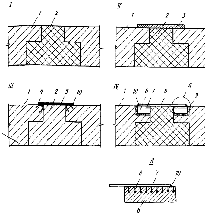
Рис. I. Конструктивные схемы стыков (I, II, III, IV) сборных железобетонных конструкций
