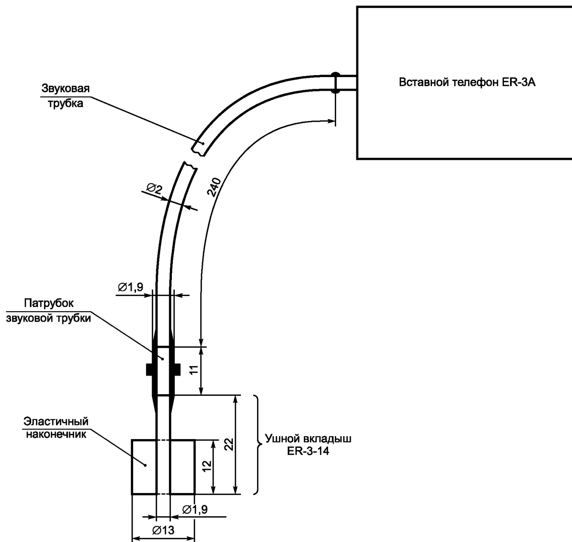
Рисунок 1 — Вставной телефон ER-3A и ушной вкладыш ER-3-14
