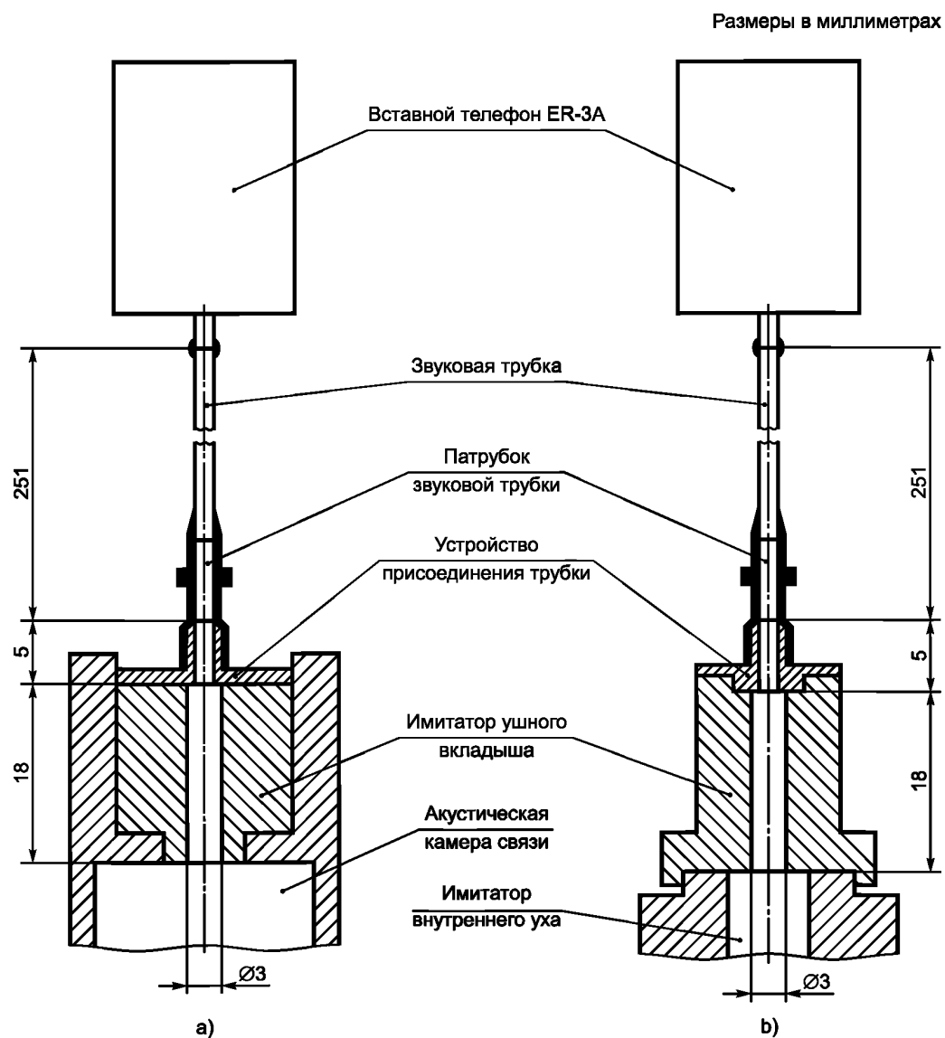
Рисунок 2 — Присоединение вставного телефона
