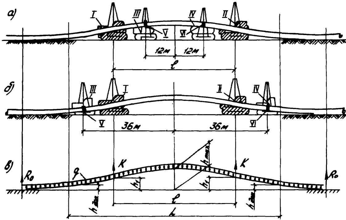
Технологические и расчетная схемы подъема трубопровода при очистке и изготовлении стыков
