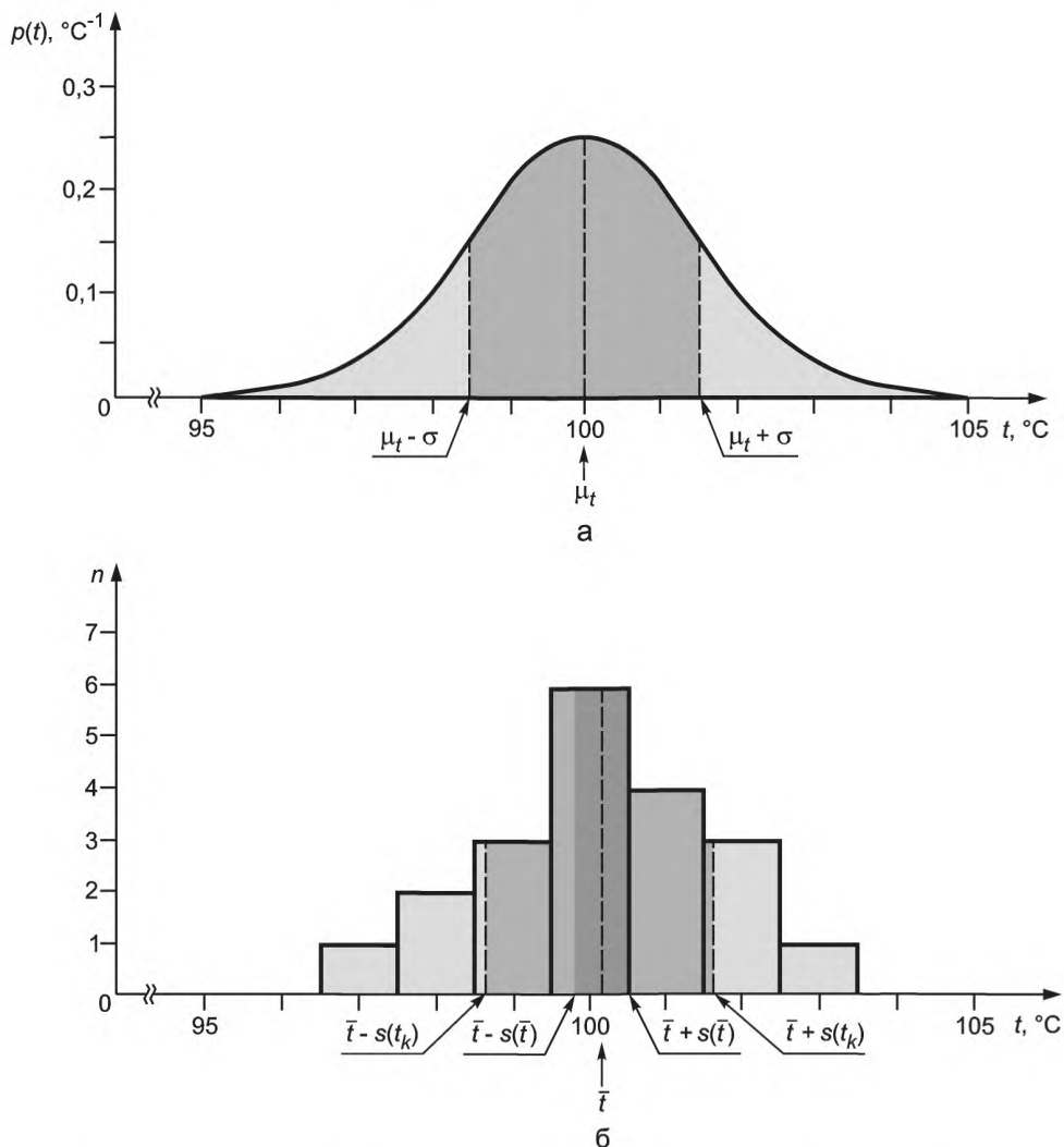
Рисунок 1 — Графическая иллюстрация оценивания стандартной неопределенности входной величины по повторным наблюдениям
