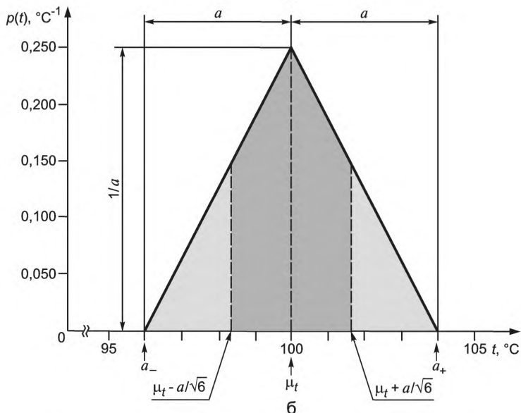
Рисунок 2 — Графическая иллюстрация оценивания стандартной неопределенности входной величины по известному закону распределения
