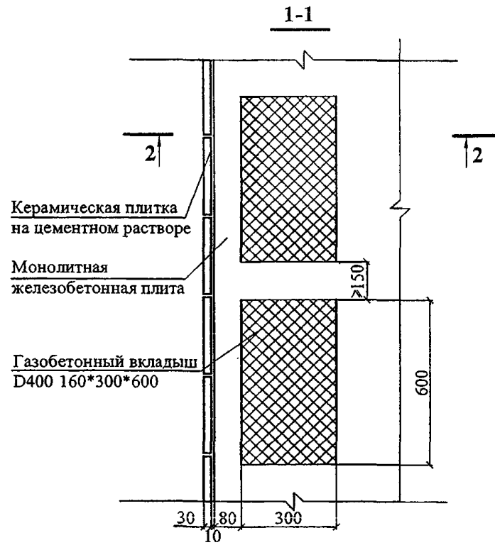
Рисунок 3. Вид по 1-1
