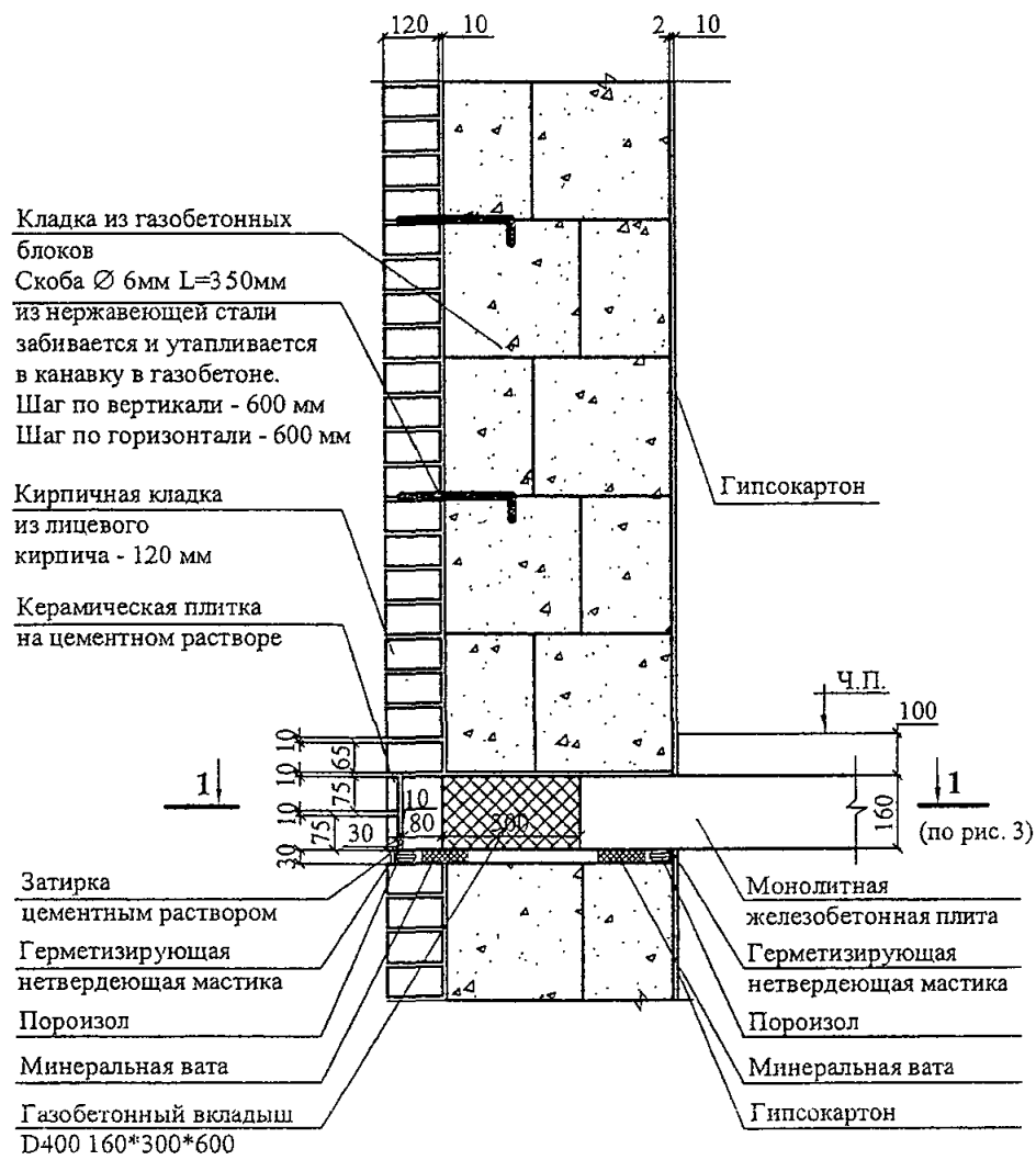
Рисунок 9. Навесная стена из кирпича и газобетонных блоков
