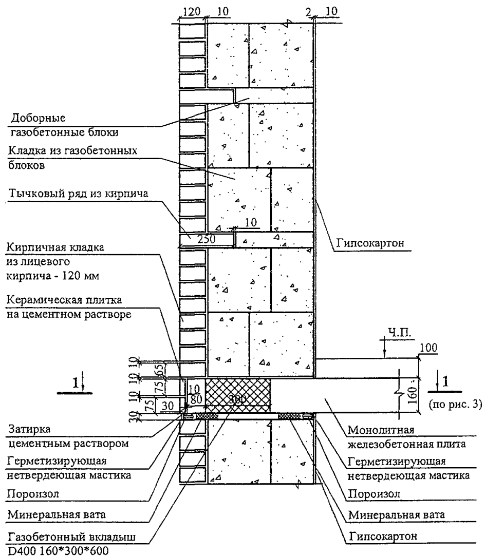
Рисунок 10. Навесная стена из кирпича и газобетонных блоков с анкеркой тычковыми рядами кирпичного облицовочного слоя
