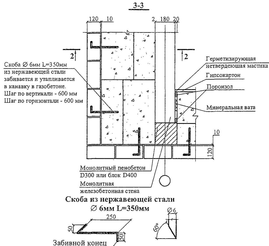
Рисунок 2. Вид по 3-3
