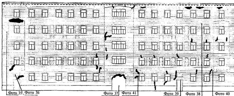
Рисунок E.1 — Пример схемы дефектов здания [87]
