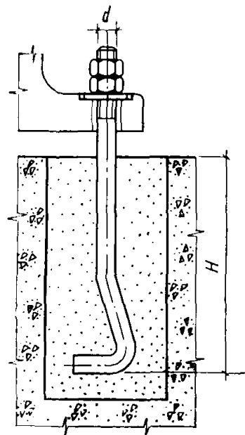
Рис. 9. Фундаментный болт, устанавливаемый в колодце с резьбой диаметром от М12 до М48 (тип 14)
