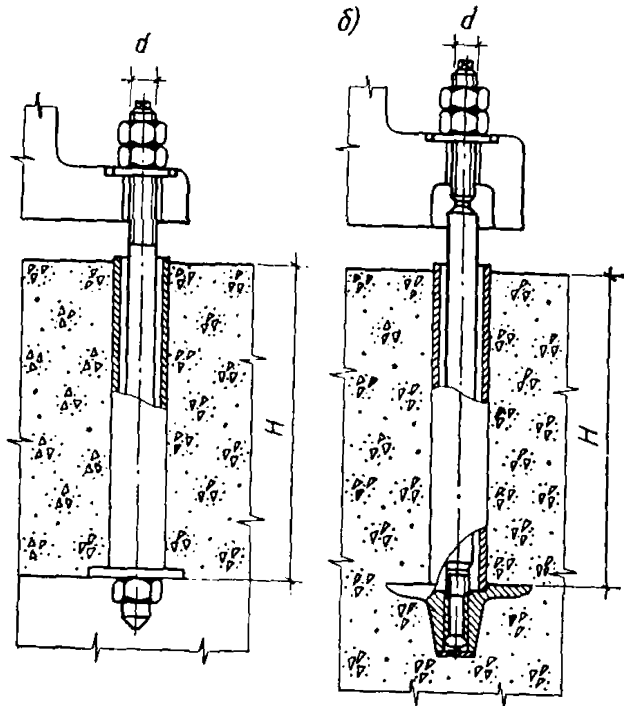
Рис. 4. Фундаментные болты с изолирующей трубой
