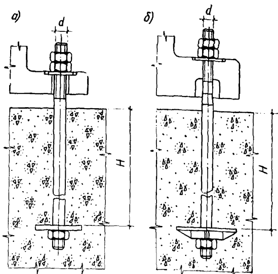
Рис. 2. Фундаментные болты с анкерными плитами
