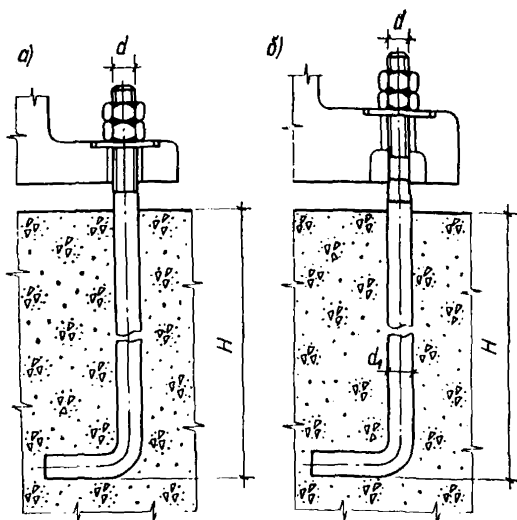
Рис. 1 Фундаментные болты с отгибом
