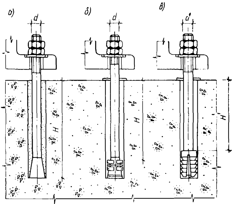
Рис. 7. Фундаментные болты конические
