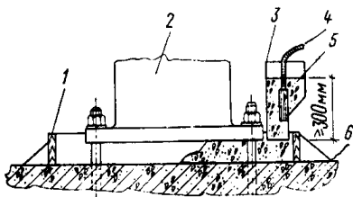
Рис. 16. Подливка оборудования с помощью лотка-накопителя
