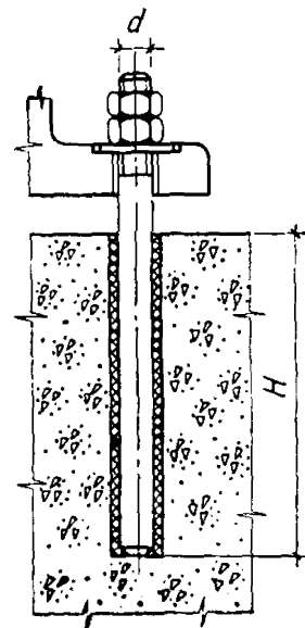
Рис. 6. Фундаментный болт на эпоксидном клею с резьбой диаметром от М10 до М100 (тип 9)
