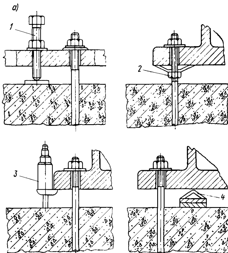
Рис. 11 Опорные элементы для выверки
