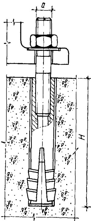
Рис. 8. Фундаментный болт составной с распорным конусом с резьбой диаметром от М12 до М24 (тип 13)
