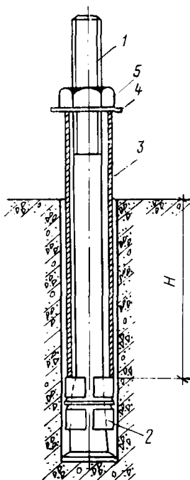
Рис. 18. Установка конического болта с распорными цангами с помощью съемной инвентарной монтажной трубки
