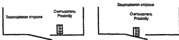
Размещение считывателей за стеной и за дверью
