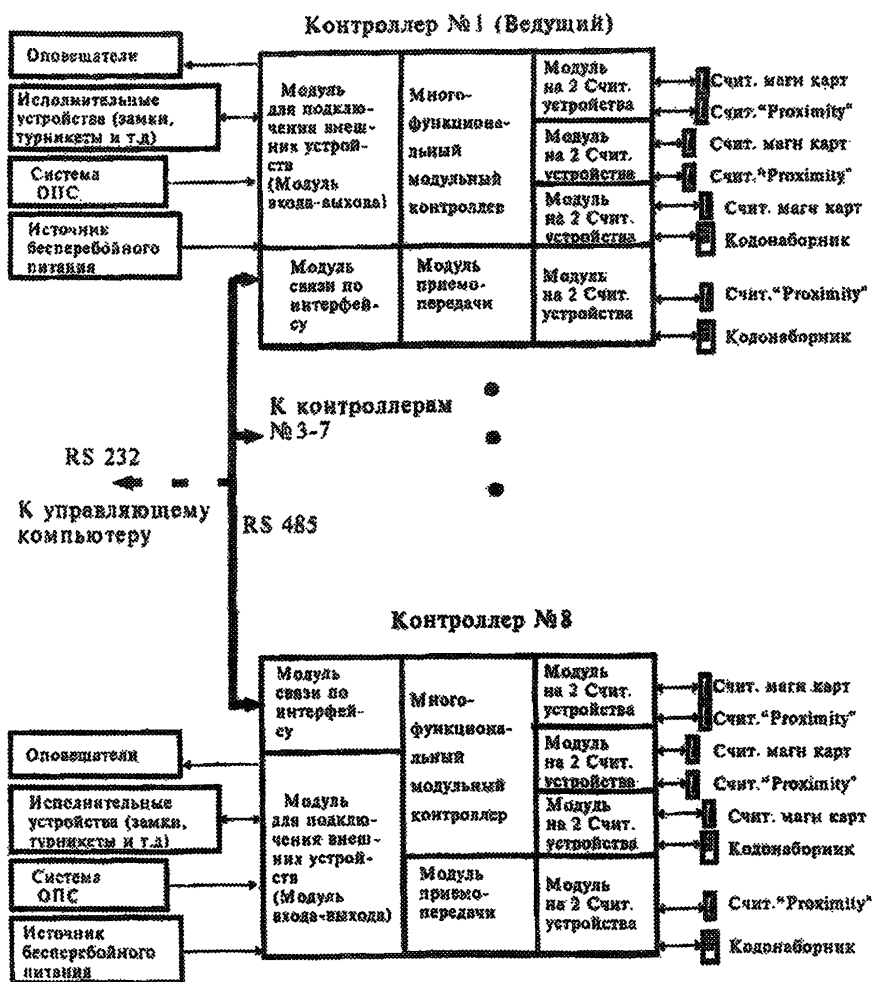
Рисунок 3 - Примерная структурная схема построения сетевой СКУД
