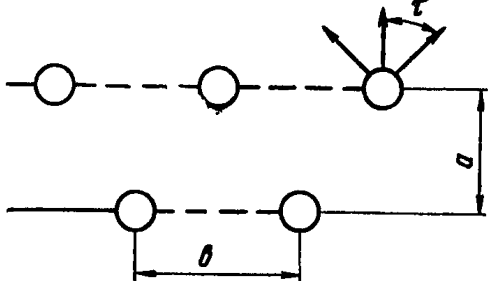
Рис. 1. Рекомендуемые схемы расположения осветительных приборов I — прямоугольное расположение мачт; II — шахматное расположение мачт; a — ширина освещаемого карьера; b — расстояние между мачтами; \tau — угол между оптическими осями
