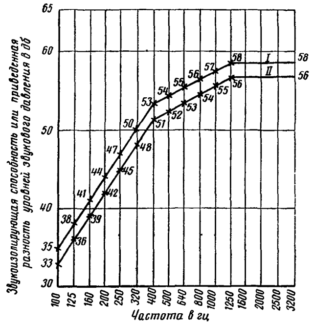
Рис. 1. Нормативные кривые звукоизолирующей способности от воздушного звука или приведенной разности уровней звукового давления I — для сравнения с кривой, полученной в лабораторных условиях; II — то же, полученной в натуральных условиях
