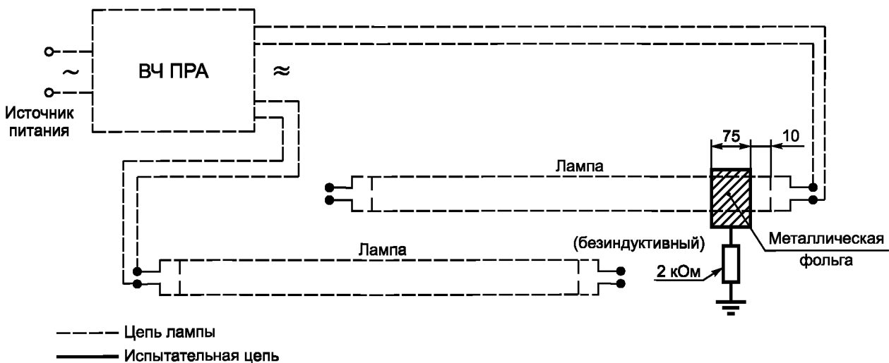
Рисунок I.1 — Испытательная установка
