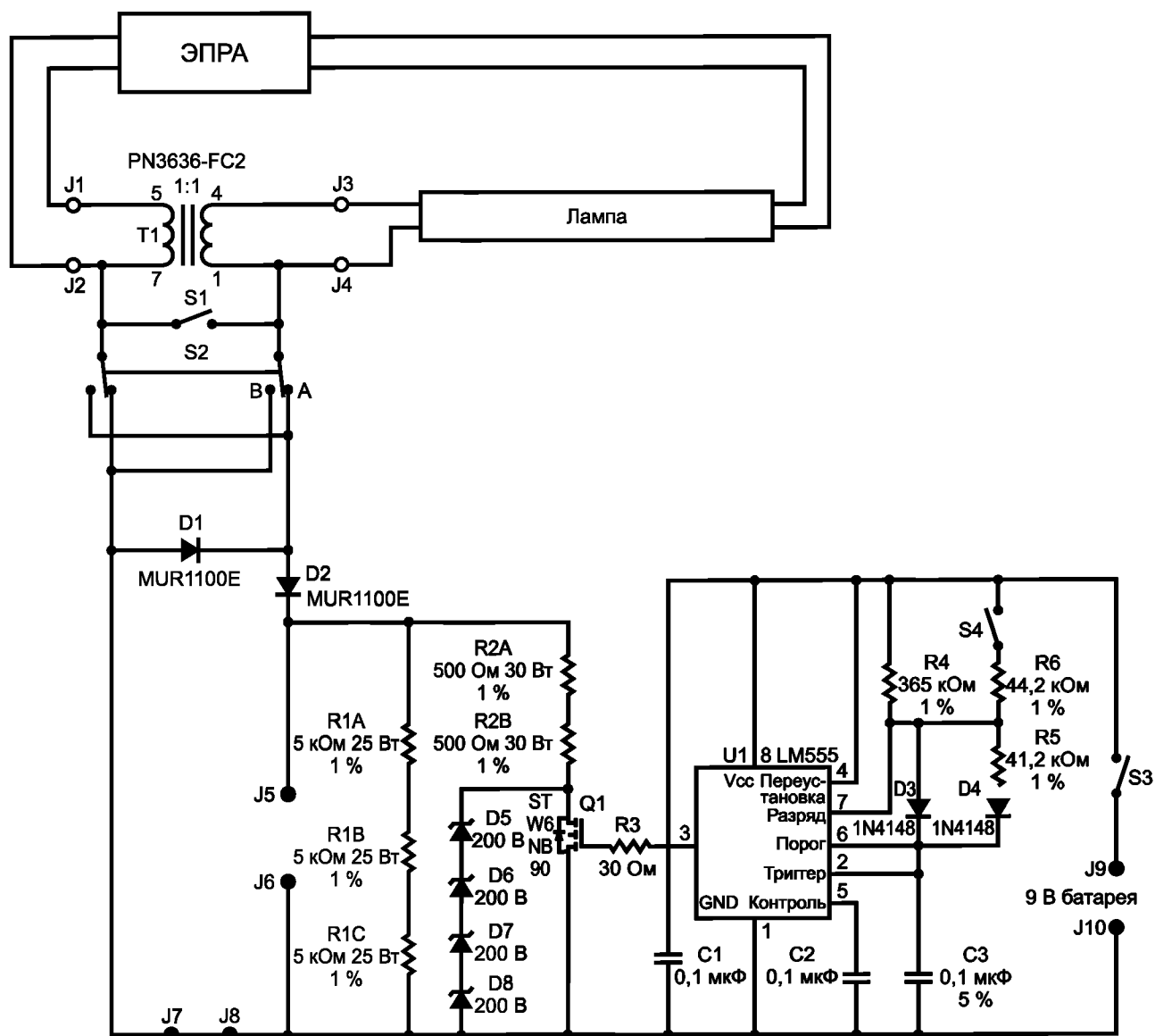
Токовый пробник постоянного тока
