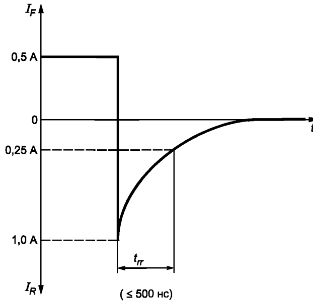
b — Время обратного восстановления диода t_{rr}
