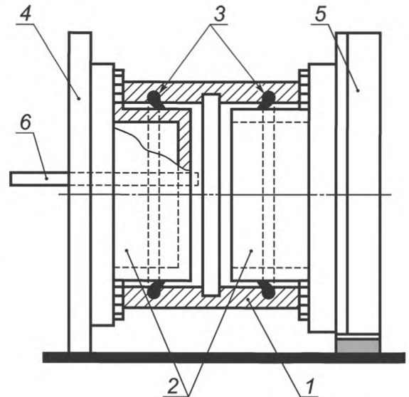
1 — муфта; 2 — оправки; 3 — кольцевые уплотнители муфты; 4 — неподвижная опора; 5 — подвижная опора; 6 — подача испытательного давления
