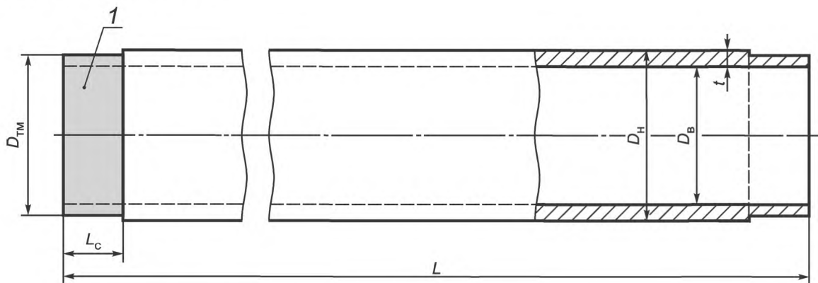
1 — калиброванная часть трубы для установки муфты; D_n — наружный диаметр; t — толщина стенки; L — длина трубы; D_{ТМ} — диаметр под муфтовое соединение (диаметр калиброванной части трубы); D_в — внутренний диаметр; L_с — длина соединения (длина калиброванной части трубы под муфтовое соединение)
