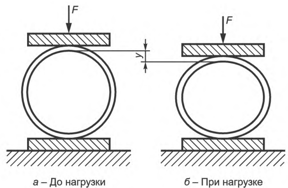
Рисунок 10 — Схема испытания на нагрузочной машине
