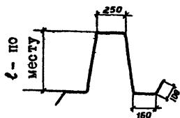
Рис. 3. Жесткий фиксатор "лягушка"
