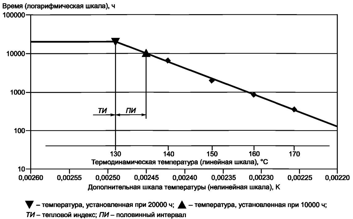
Рисунок А.2 — График теплостойкости
