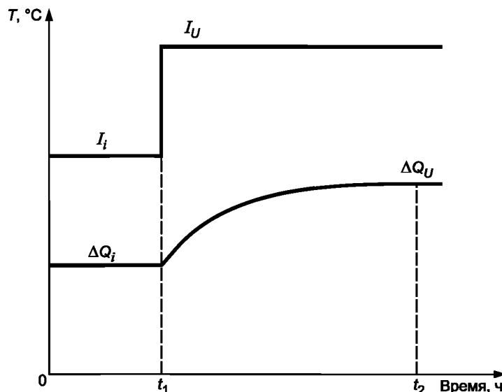
Верхняя кривая: начальная и максимальная нагрузки. Нижняя кривая: рост температуры свыше температуры окружающей среды
