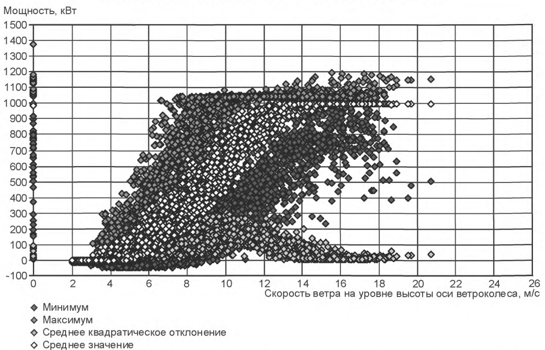
Рисунок 2 — Пример представления баз данных А и В: графики разбросов характеристик мощности в эксперименте, выборка которого проведена с частотой 1 Гц (средние значения получены усреднением за 10 мин)
