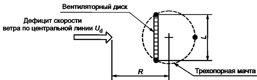
Рисунок G.7 — Представление трехопорной решетчатой мачты с указанием дефицита скорости ветра по центральной линии; представление вентиляторного диска мачты с шириной фронтальной поверхности L и расстоянием R от центра мачты до точки наблюдения
