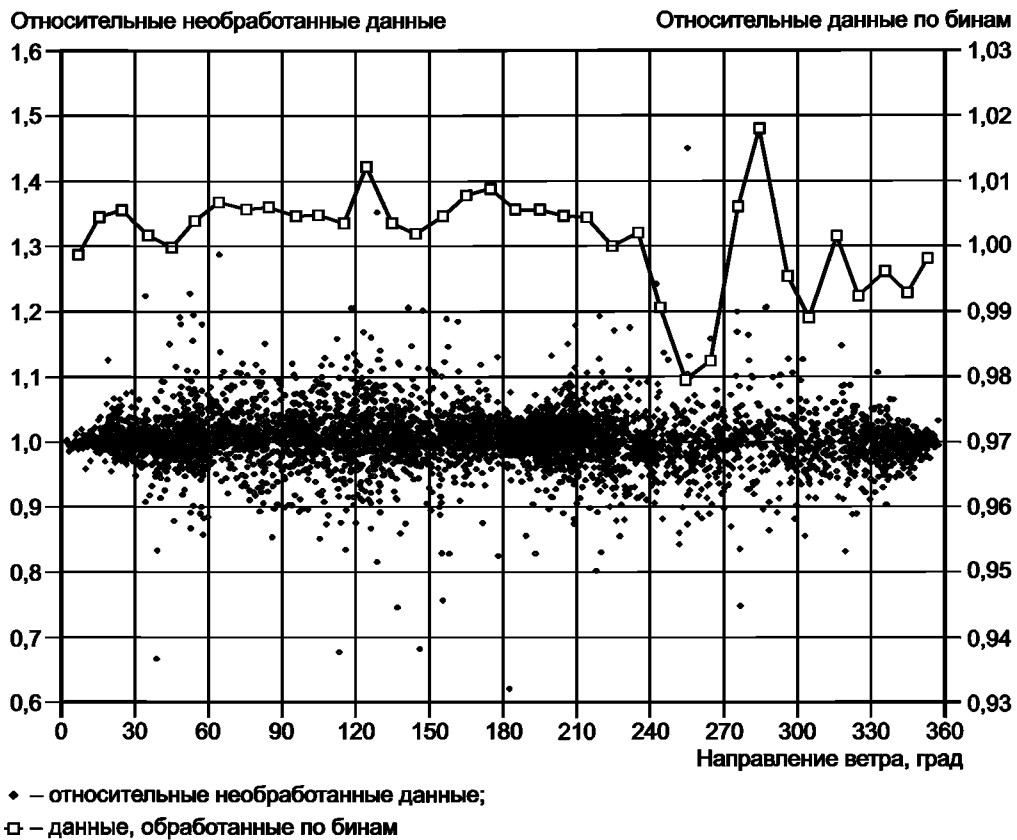
Рисунок 5 — Пример представления калибровки площадки (эффективные секторы только от 20° до 30°, от 40° до 60°, от 160° до 210° и от 330° до 350°)
