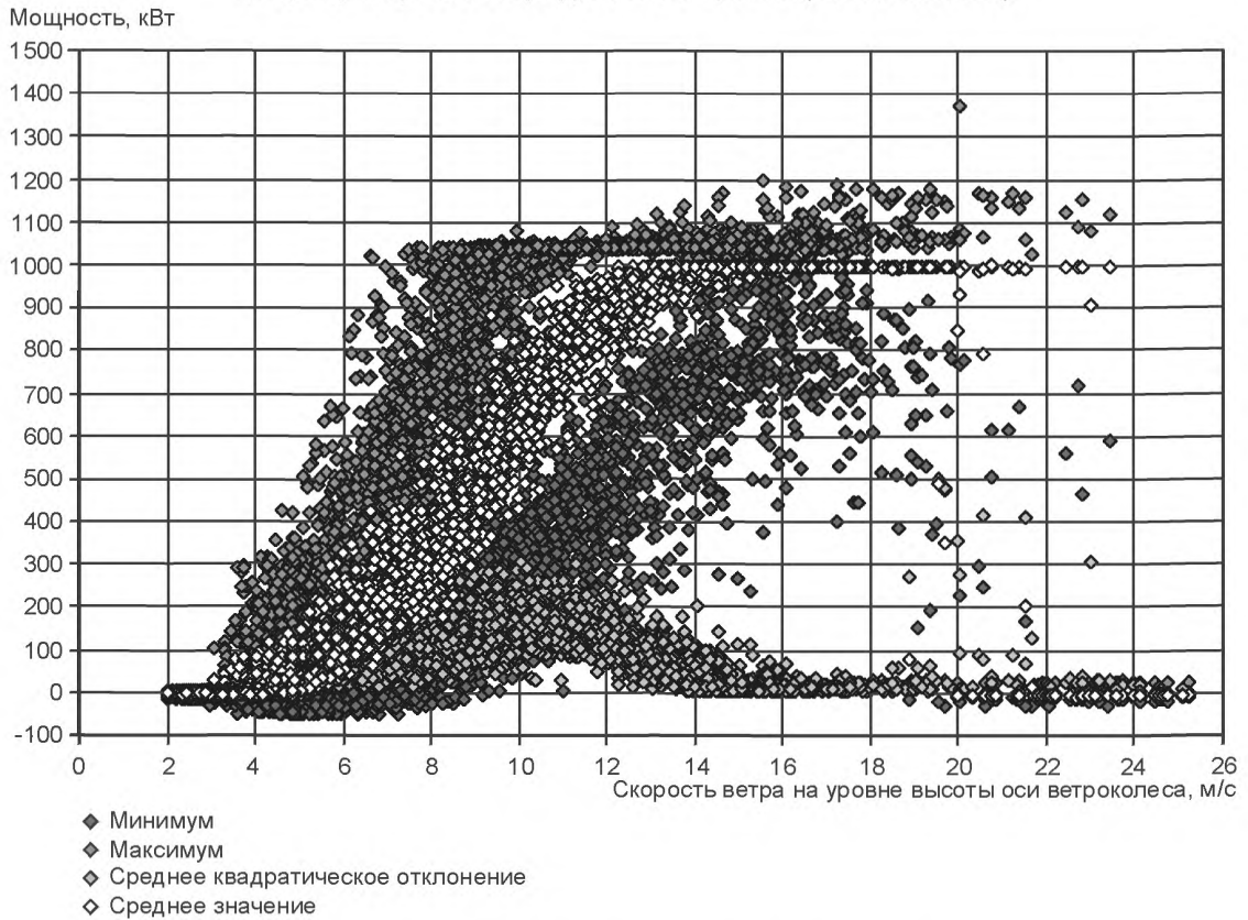
График разброса генерируемой мощности (база данных В)
