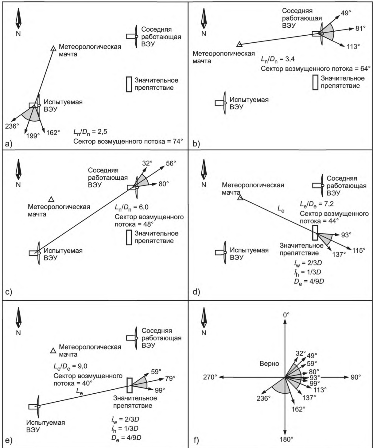
Рисунок А.2 — Пример секторов, которые необходимо исключить из-за воздействия турбулентного следа на испытуемую ВЭУ в результате влияния соседней работающей ВЭУ и значительного аэродинамического препятствия
