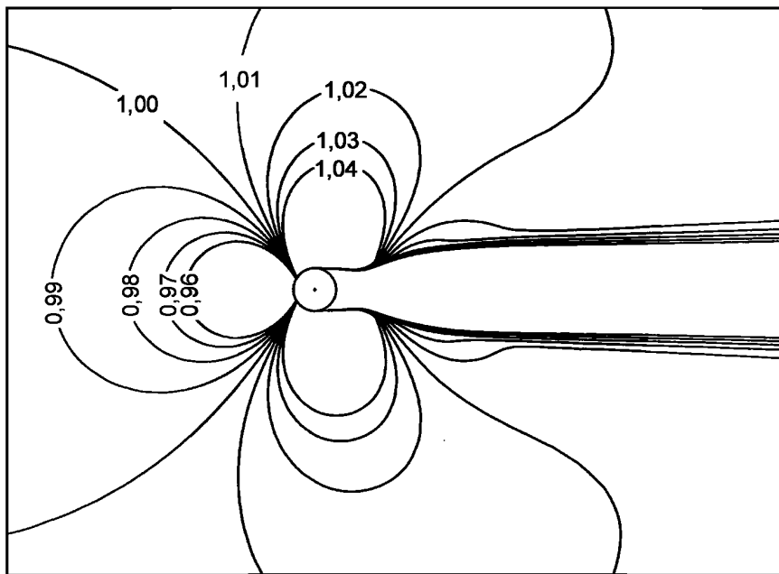
Рисунок Г.5 — Поле распределения скоростей обтекания трубчатой мачты, нормализованное невозмущенным полем скоростей воздушного потока (слева); компьютерный расчет двумерных уравнений Навье — Стокса
