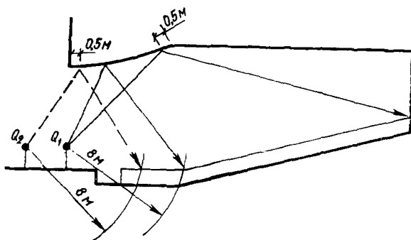
Рис. 3. Звукоотражатель в передней части потолка
