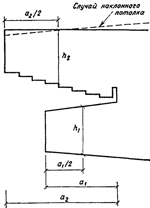
Рис. 13. Надбалконные и подбалконные пазухи
