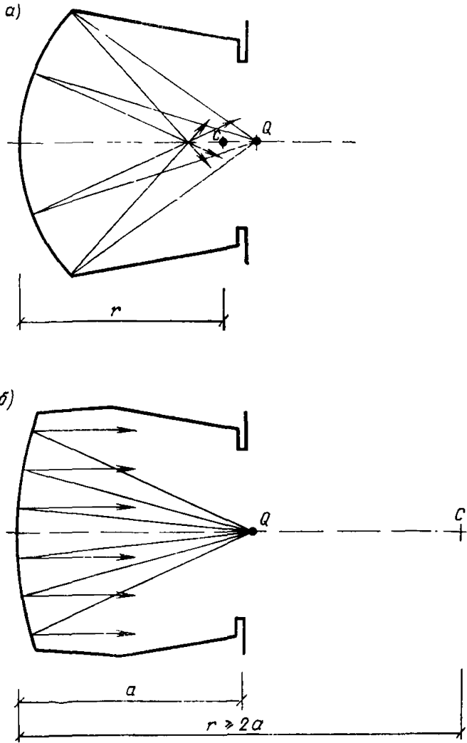
Рис. 9. Отражения звука от вогнутой задгнутой стены
