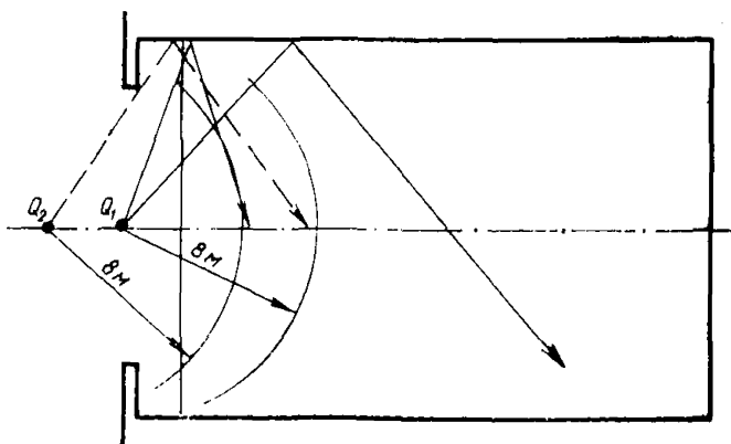
Рис. 6. Распределение отражений при параллельных боковых стенах
